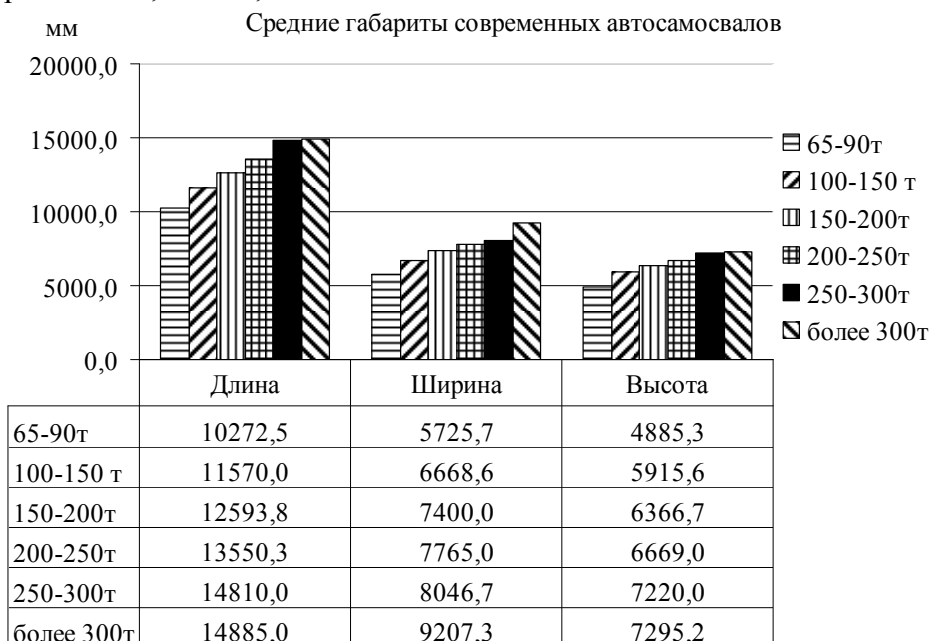
Рис. 3. Гистограмма средних основных рабочих параметров большегрузных автосамосвалов
