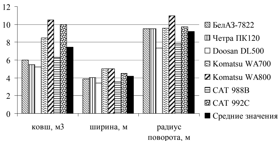
Рис. 2. Гистограмма рабочих параметров современных погрузчиков
