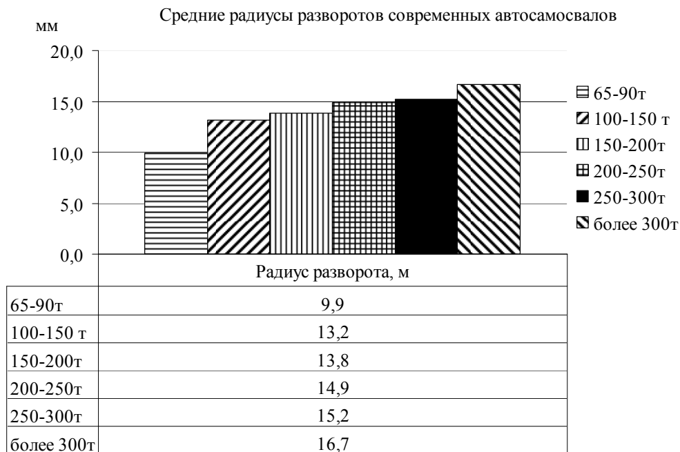
Рис. 4. Гистограмма средних радиусов разворотов современных большегрузных автосамосвалов
