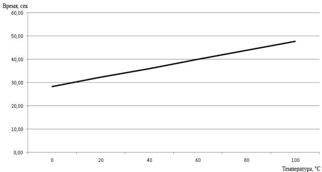
Рис. 3. Статическая характеристика теплового объекта
