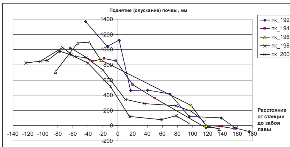
Рис. 8. Сводный график опускания (поднятия) почвы 163-го сборного штрека
