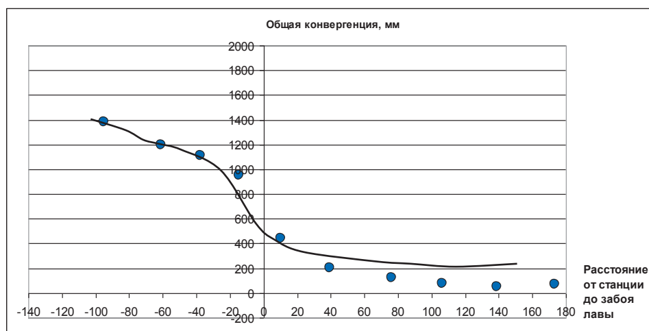
Рис. 9. Сглаженный график конвергенции 159-го и 163-го сборных штреков
