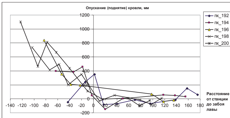
Рис. 7. Сводный график опускания (поднятия) кровли 163-го сборного штрека
