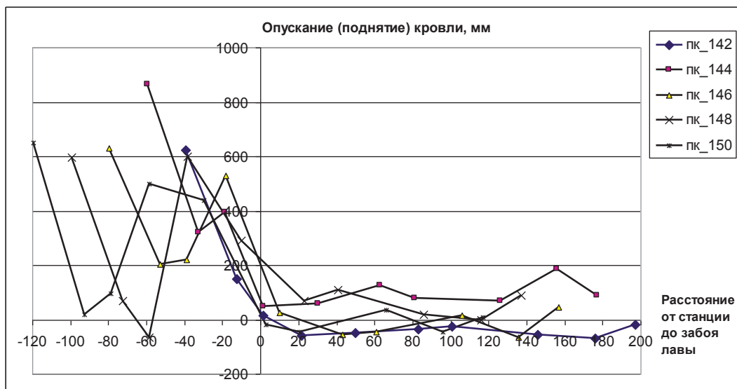
Рис. 4. Сводный график опускания (поднятия) кровли 159-го сборного штрека
