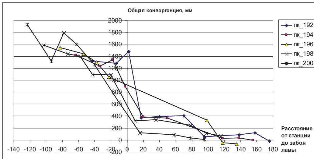
Рис. 6. Сводный график общей конвергенции 163-го сборного штрека
