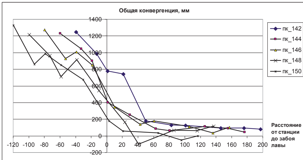
Рис. 3. Сводный график общей конвергенции 159-го сборного штрека
