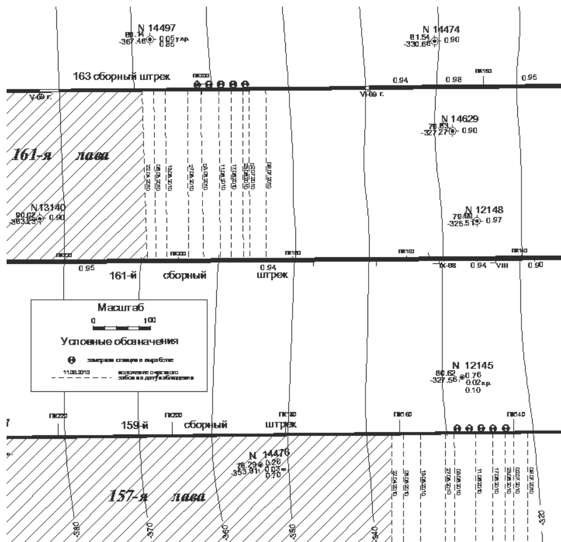
Рис. 1. Выкопировка из плана горных выработок.
