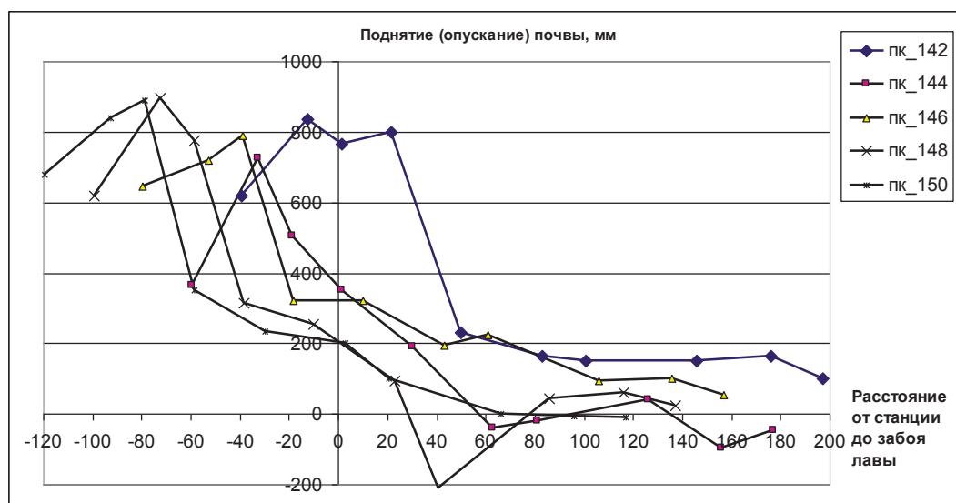
Рис. 5. Сводный график опускания (поднятия) почвы 159-го сборного штрека
