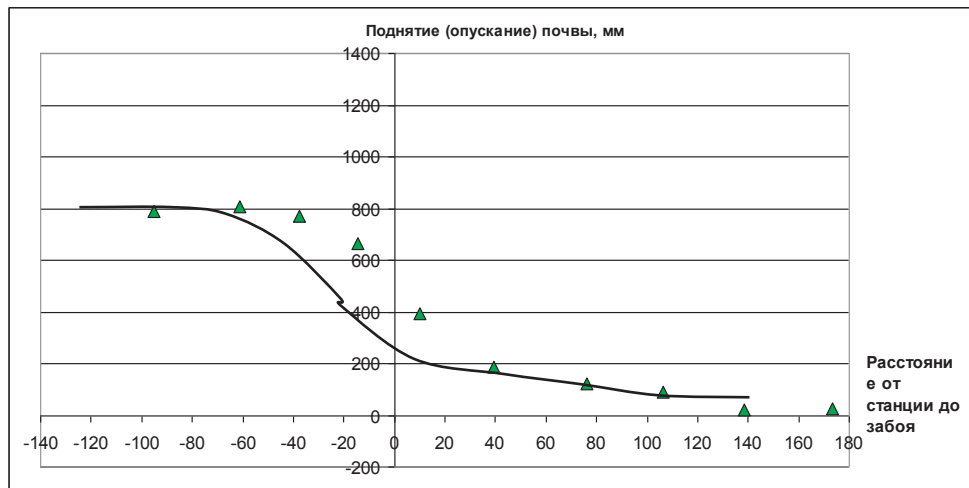
Рис. 11. Сглаженный график поднятия почвы 159-го и 163-го сборных штреков
