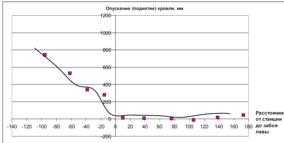
Рис. 10. Сглаженный график опускания кровли 159-го и 163-го сборного штреков
