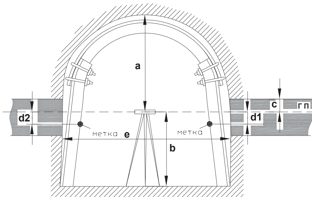
Рис. 2. Схема маркшейдерских замеров на наблюдательной станции
