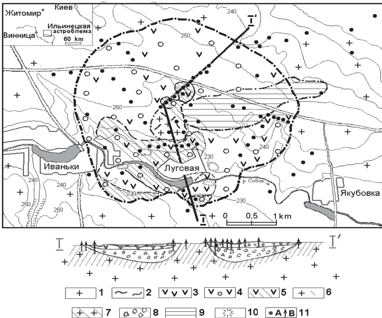
Рис.1. Схематична геологічна карта і розріз Іллінецької астроблеми
