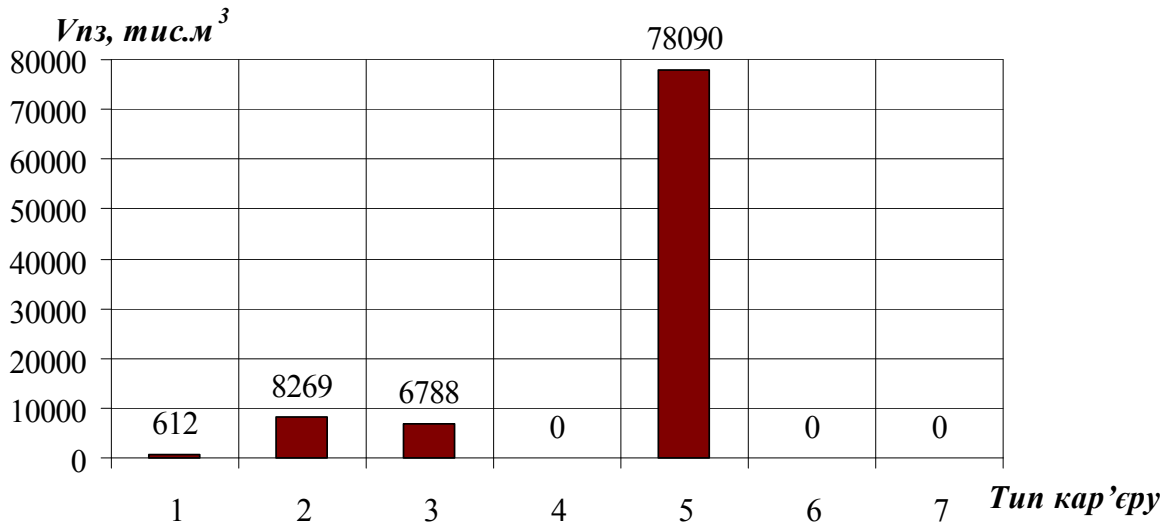
Рис. 4. Об'єм природжених запасів корисної копалини на базових кар'єрах (базові кар'єри 4, 6 і 7 типів з видобутку пластових родовищ флюсодоломітної сировини відпрацьовуються до проектної глибини КПЧ)
