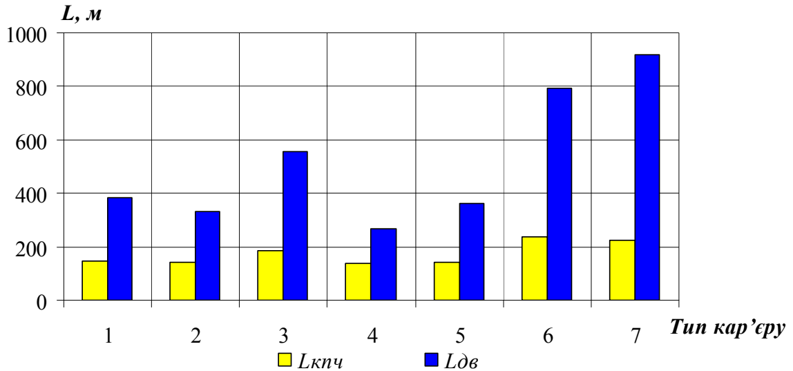
Рис. 3. Параметри довжини КПЧ по поверхні ( L_{КПЧ} ) та довжина ділянки дна КПЧ, зайнята під внутрішні відвали ( L_{ов} )
