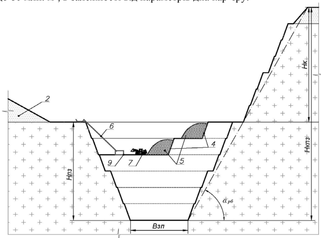
Рис. 2. Схема відпрацювання природних запасів корисної копалини (розріз А-А рис. 1, б ): 2, 4-7, 9 – див. рис. 1
