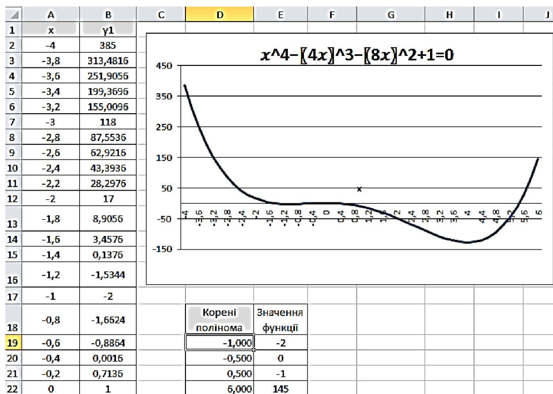
Рис. 2.3. Графік поліному x^4 - 4x^3 - 8x^2 + 1 = 0
