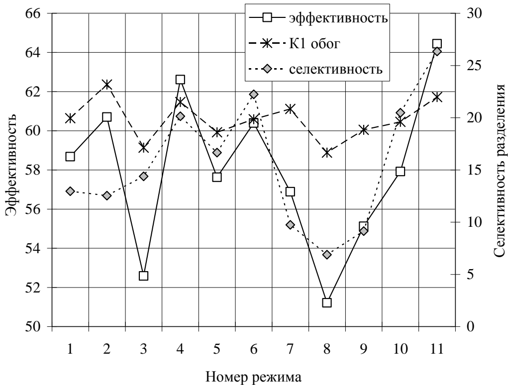
Рис. 2. Технологические показатели обогачення угільного шламу на концентраційному столі СКО-5x2 в польових умовах
