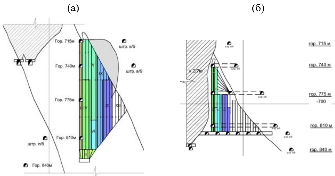
Рис.1. Оптимизация параметров камерной системы разработки при отработке запасов руд на контакте с неустойчивыми вмещающими породами: (а) камерная система разработки с наклонным днищем и выпуском руды на виброполки; (б) камерная система разработки с плоским днищем и погрузкой руды ПДМ
