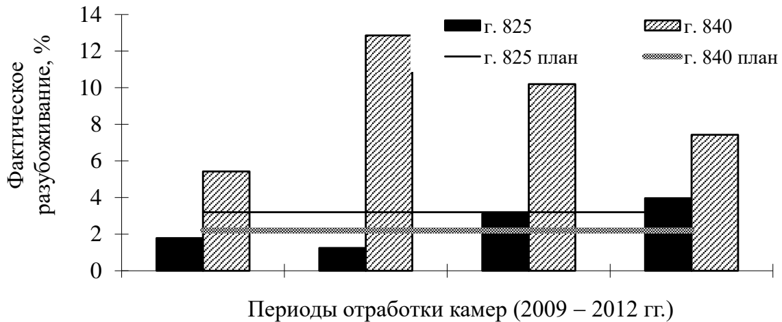
Рис. 5. Эффективность управления качеством добытой руды из камер
