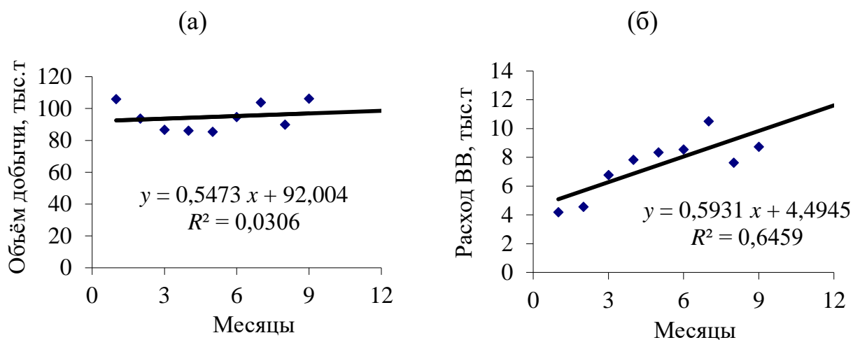
Рис. 4. Прогноз объемов добычи полезного ископаемого (а) и расхода ВВ (б) при используемой технологии выпуска на гор. 840 м
