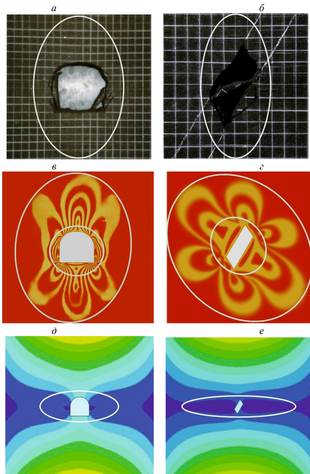
Рис. 1. Результаты выявления энергетических зон при моделировании подготовительных ( a , в , д ) и очистных ( б , г , е ) выработок на эквивалентных ( a , б ), оптико-поляризационных ( в , г ) и электропроводных ( д , е ) материалах: эллиптические линии вокруг выработок – границы зон, где напряжения приближаются к \gamma H
