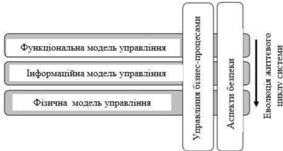
Рисунок 1.5 – Архітектура управління мережі NGN
