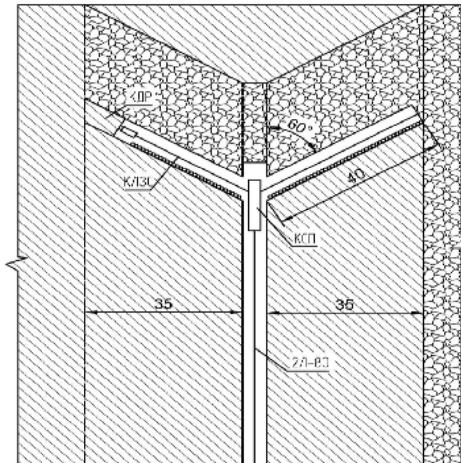
Рис. 2.1. Схема діагонального розташування виїмкових заходок
