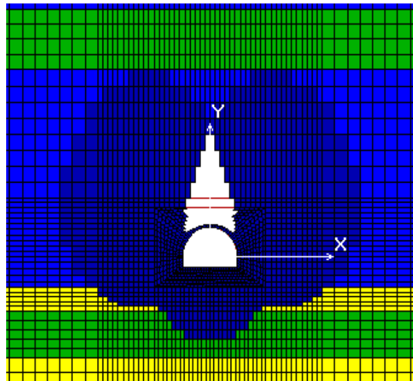
Рис. 5. Численное решение задачи о вывалообразовании в условиях вертикальной трещиноватости окружающего породного массива [19]
