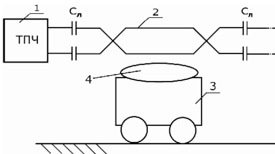
Рис. 1. Принципиальная схема транспорта с индуктивной передачей энергии: 1 – ТПЧ; 2 – тяговая сеть; 3 – подвижной состав; 4 – энергоприемник; C_{л} – компенсирующий конденсатор
