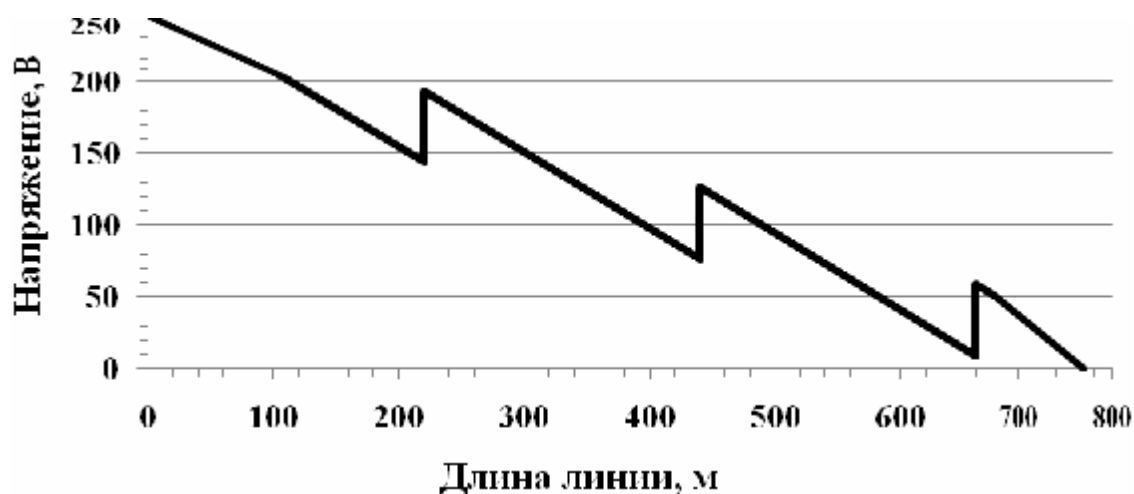
Рис. 3. График распределения напряжений вдоль тяговой сети
