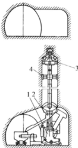
Рис. 4.2. Комбайн 1КВ-1: 1 – комбайн; 2 – шламочистковий пристрій; 3 – робочий інструмент; 4 – опорний ліхтар
