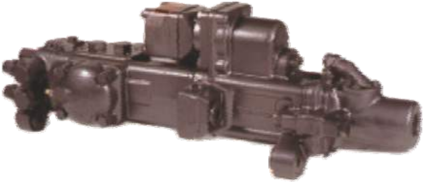
Рис. 1.46. Загальний вигляд гідравлічних перфораторів HL600 і HL600S
