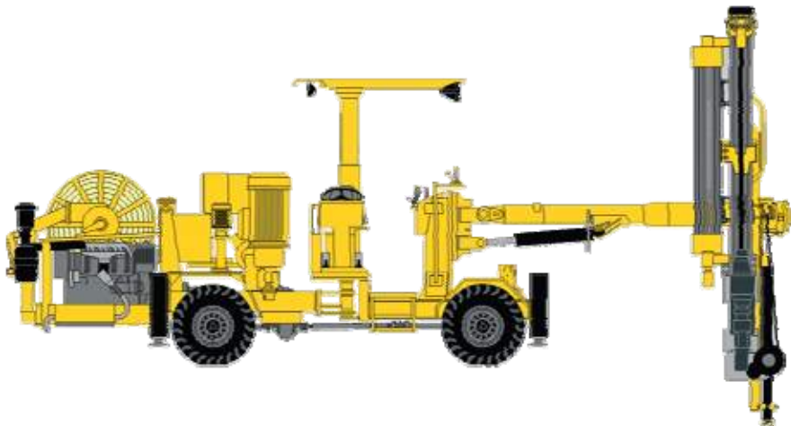
Рис. 3.10. Загальний вигляд бурового верстата Simba H257
