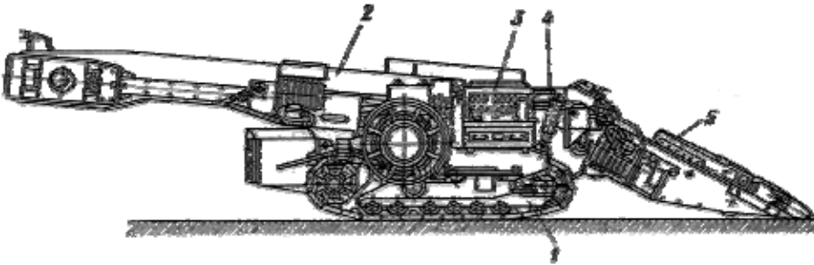
Рис. 5.9. Загальний вигляд і основні вузли вантажної машини ПНБ-4: 1 – гусеничний хід; 2 – скребковий конвеєр; 3 – електроустаткування; 4 – гідросистема; 5 – виконавчий орган
