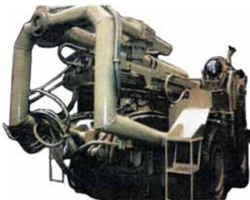
Рис. 3.7. Загальний вигляд верстата бурового самохідного БУ-85С
