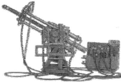
Рис. 3.4. Загальний вигляд верстата шарошечного буріння БШ-145
