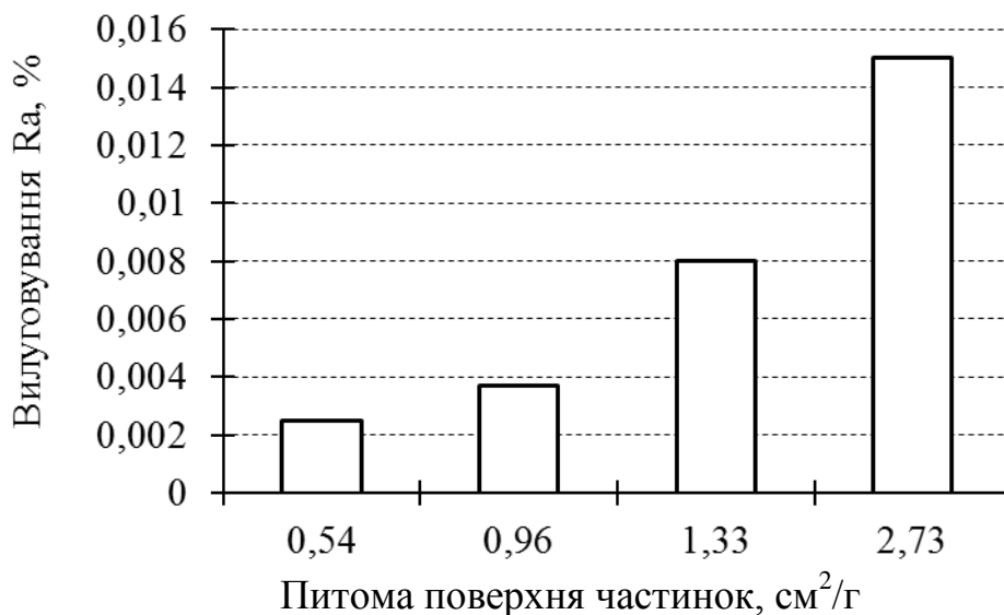
Рис. 5.1. Діаграма залежності вилугування радію від дисперсності породи
