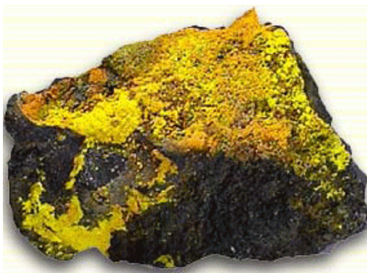
Рис. 2.3. Уранові черні
