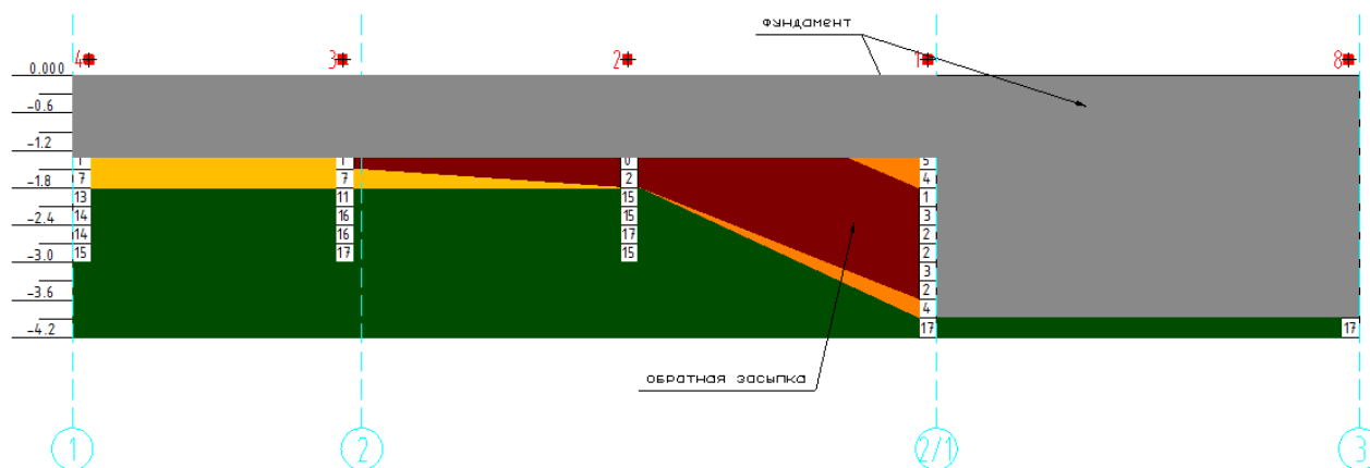
Рис. 1. Геологический разрез, построенный по результатам динамического зондирования основания
