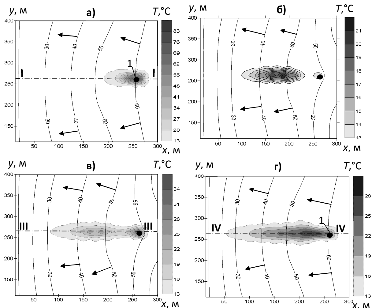
Рисунок 4 – Распределение уровня подземных вод (изогипсы) и их температуры (оттенки серого цвета) в водоносном горизонте, залегающем над угольным пластом при его отработке способом ПСУ: а), б) – по окончании сжигания угля ( t = 30 сут) соответственно на высоте 1 и 3 м от водоупора; в) при завершении отбора нагретых вод ( t = 180 сут); г) после последующе-
