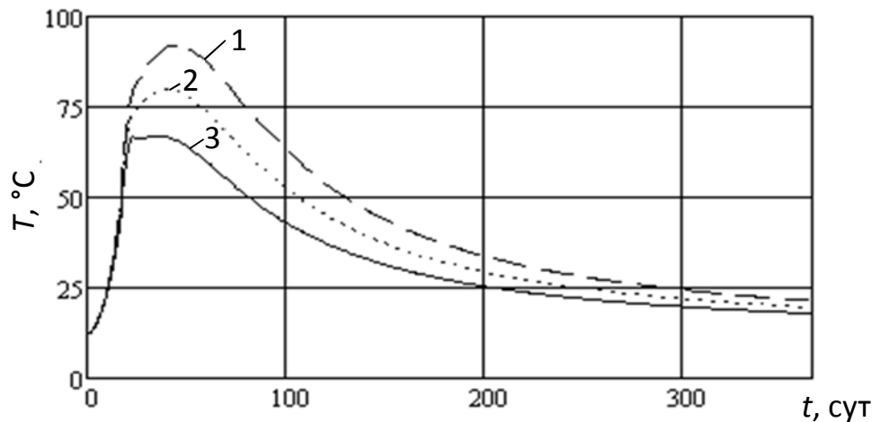
Рисунок 3 – Изменение температуры пород водоносного горизонта непосредственно над кровлей сжигаемого угольного пласта с углом падения 10°: 1 – V=0,92 \text{ м/сут} (природный режим фильтрации); 2 – V=1,13 \text{ м/сут} (закачка воды в пласт); 3 – V=1,45 \text{ м/сут} (отбор подземных вод)
