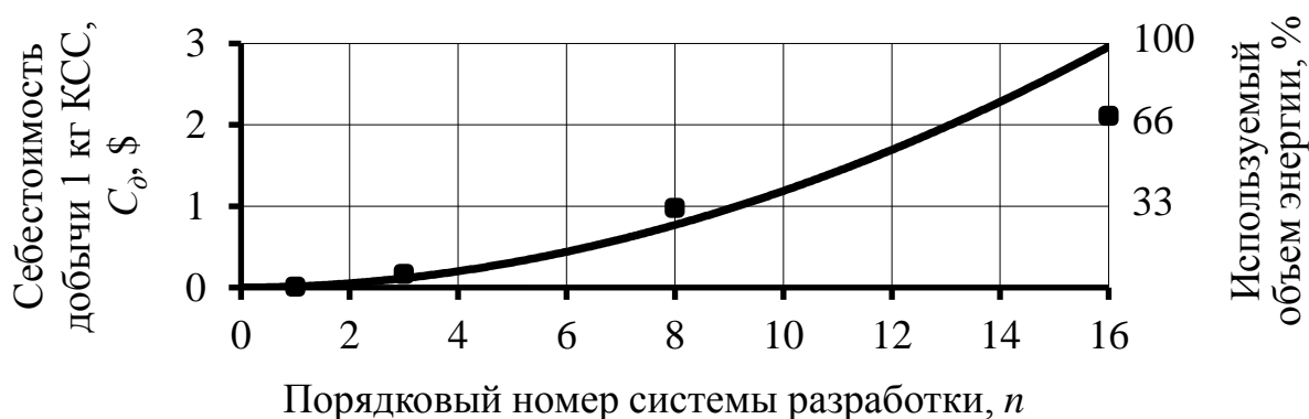
Рис. 1. Себестоимость добычи 1 кг КСС по вариантам систем разработки
