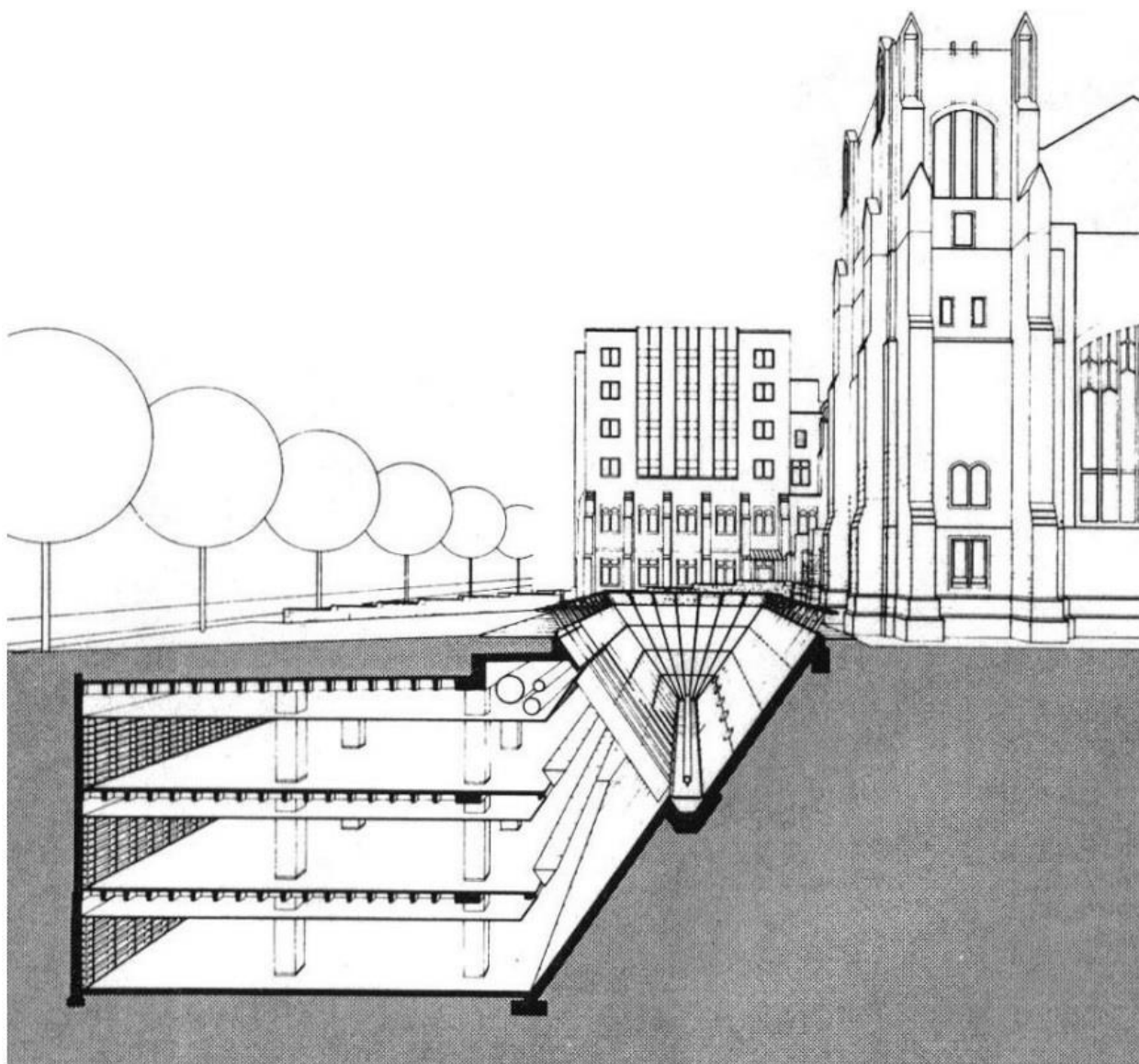
Рис. 3. Розріз прибудови до будівлі юридичної бібліотеки університету штату Міннесота
