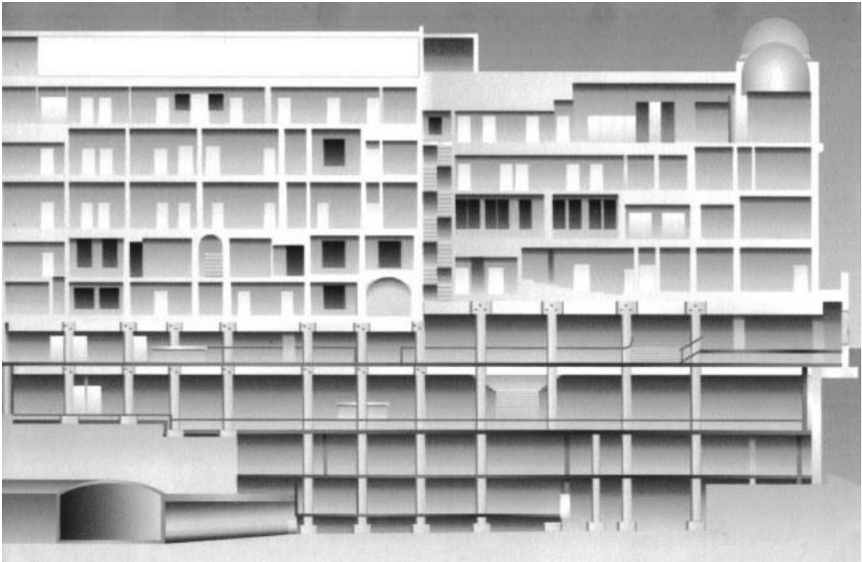
Рис. 1. Розріз по будівлі готелю Nikolajeff House і комунікаційному тунелю
