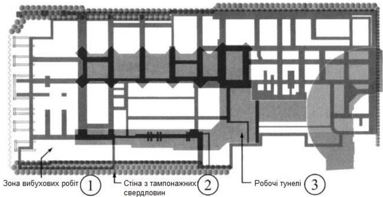
Рис. 2. План підвалу готелю Nikolajeff House
