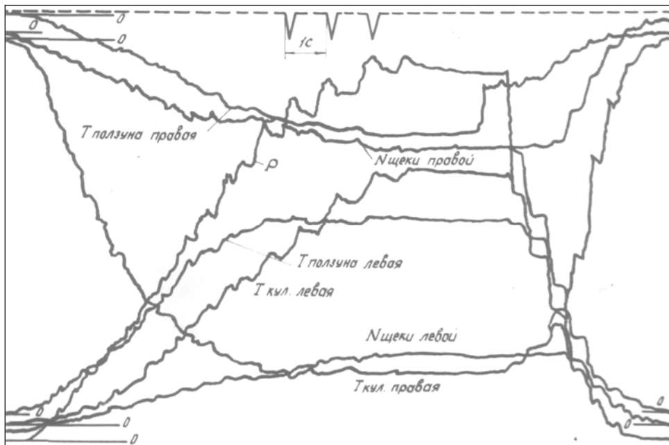
Рисунок 2 - Осциллограмма испытаний
