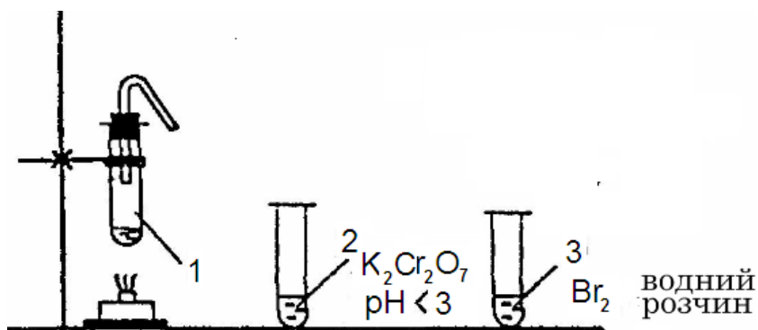
Рис. 1. Схема проведення дослідів добування насичених та ненасичених вуглеводнів, їх бромовання
