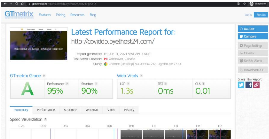
Рис. 2.9. Тестування у сервісі GTmetrix
