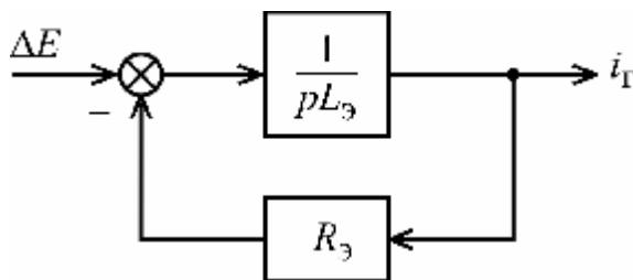
Рис. 2. Структурная схема регулирования тока I_r
