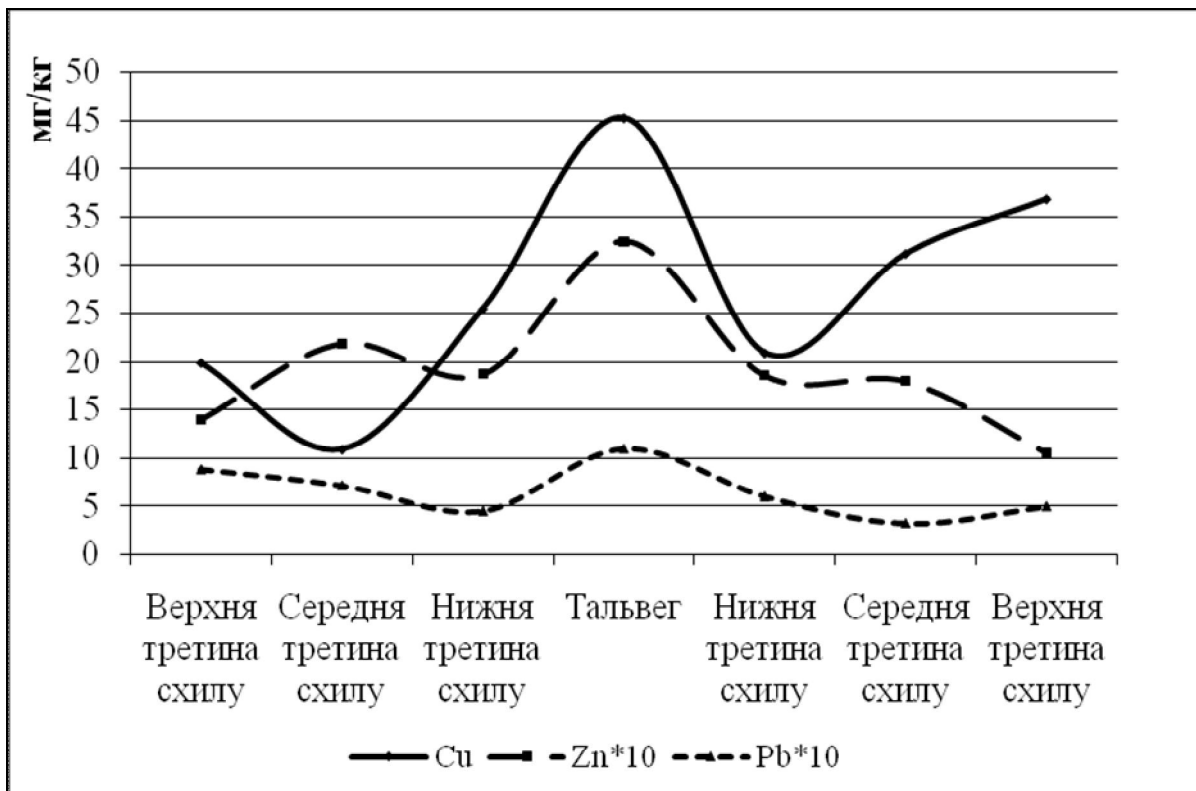
Рис. 1. Розподіл свинцю ( n \cdot 10 ), міді та цинку ( n \cdot 10 ) у ґрунтах в профілі балки Самишиної (захід – схід)
