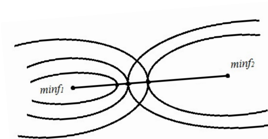
Рис. 2.10. Криві рівного рівня для функцій f_1(x_1, x_2) і f_2(x_1, x_2) .
