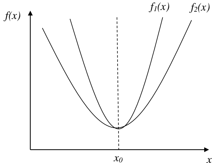
Рис. 2.8. Багатокритерійна оптимізація з не суперечливими критеріями
