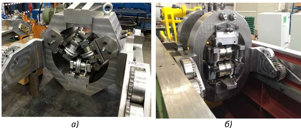
Рис. 5 – Общий вид стана ХПТ-30: а) трехвалковый; б) двухвалковый
