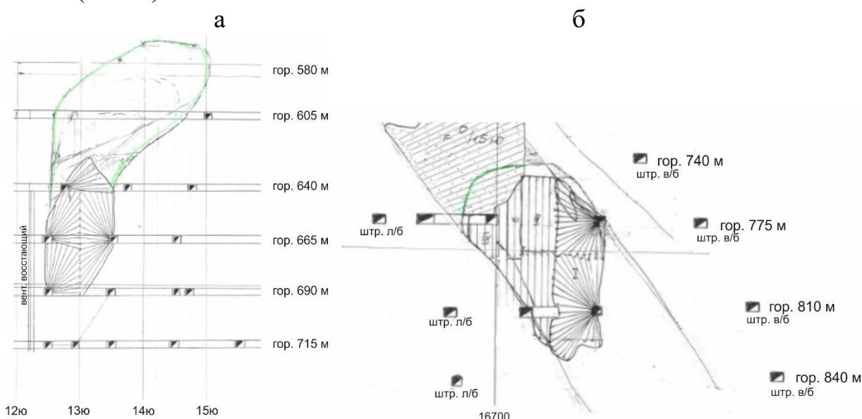
Рис. 2. Обрушение искусственного массива с бортов и кровли в очистное пространство камеры: а - 00/13ю (вид по простиранию залежи); б – 1/15ю (вид вкрест простирания залежи)
