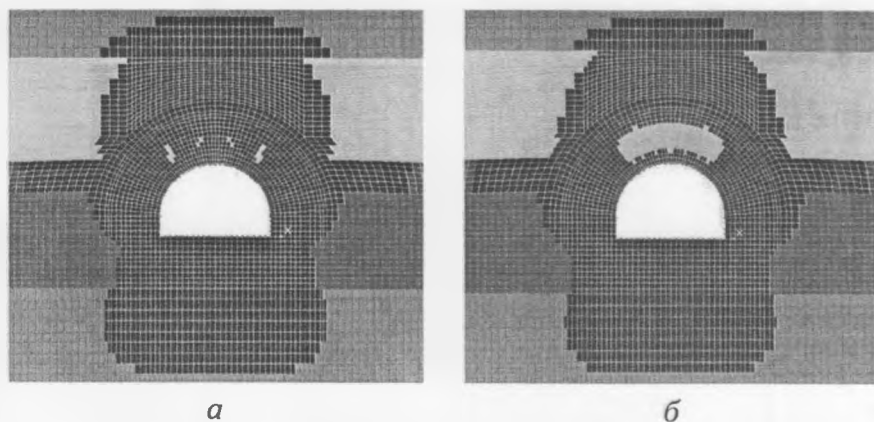
Рис. 3. Прилегающая к выработке зона разрыхления и зоны упрочненных пород при креплении выработки: а – арочной крепью и дополнительно четырьмя анкерами длиной 2,2 м; б – арочной крепью и дополнительно семью анкерами длиной 2,2 м.
