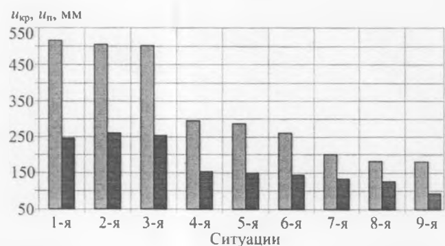
Рис. 2. Изменения смещений кровли u_{кр} и подошвы u_{п} при разном креплении наклонной выработки.
