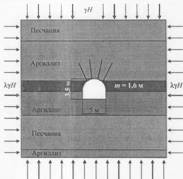
Рис. 1. Расчетная схема к решению задачи определения рациональной плотности анкерования наклонных выработок тремя – девятью анкерами длиной 2,2 м.
