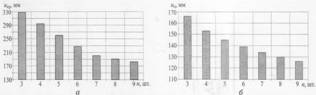
Рис. 5. Изменение в зависимости от количества n анкеров: а – смещения кровли; б – смещения подошвы.
