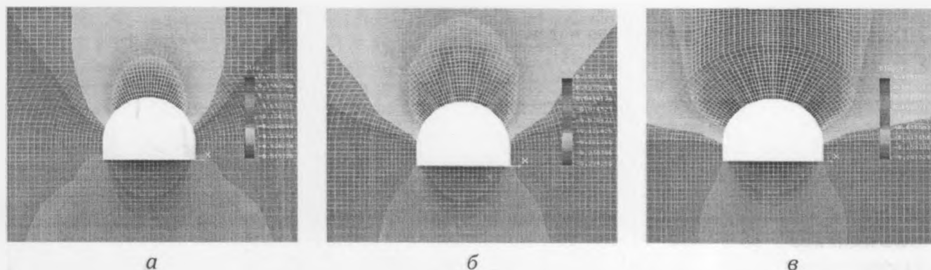
Рис. 4. Картина распределения полных перемещений: а – при незакрепленной выработке; б – при креплении выработки арочной крепью и дополнительно четырьмя анкерами длиной 2,2 м; в – при креплении выработки арочной крепью и дополнительно семью анкерами длиной 2,2 м.
