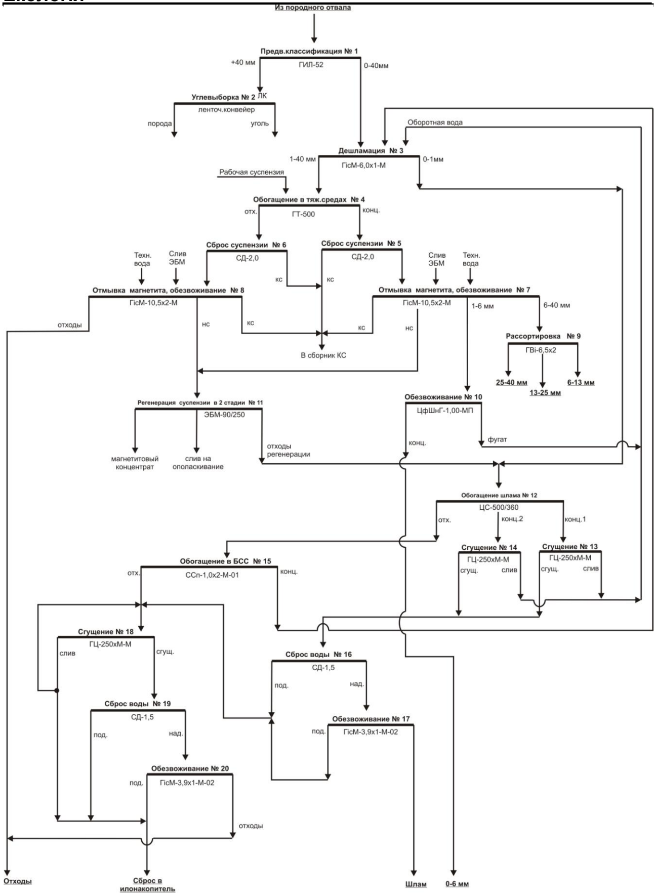
Технологическая схема переработки породного отвала
