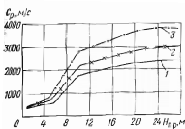
Рис. 1. Зміна швидкості поширення поздовжніх хвиль напружень в залежності від глибини свердловини: 1 – діорити; 2 – гранодіорит-порфіри; 3 – вапняки
