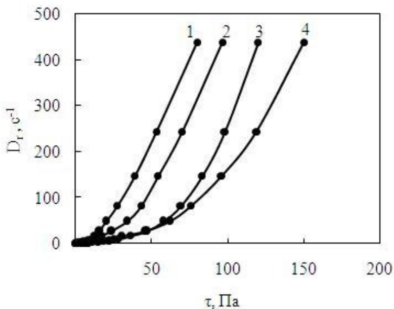
Рис. 3. Кривые течения ВУС на основе бурого угля ( C_T=55\% ) в присутствии ЛСТНа ( C_d=1\% ) с молекулярной массой: 1 – M=1000 ; 2 – M=10000 ; 3 – M=50000 ; 4 – M > 50000
