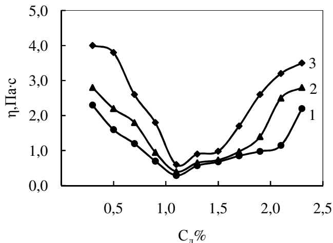
Рис. 2. Влияние концентрации ЛСТНа в сочетании с NaOH на реологические свойства ВУС ( C_T=50\% ) на основе бурого угля: 1 – NaOH:ЛСТНа = 1:9; 2 – NaOH:ЛСТНа = 1:4; 3 – NaOH:ЛСТНа = 3:7
