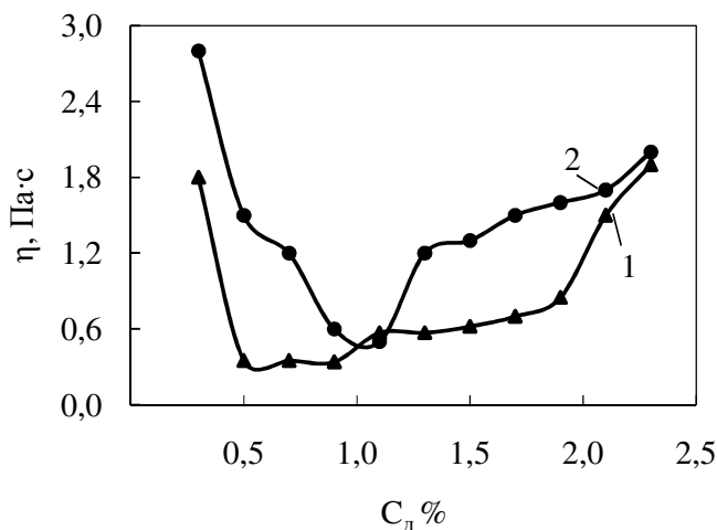
Рис. 1. Влияние концентрации ЛСТНа на реологические свойства ВУС на основе бурого угля при C_T равной: 1 – 45%; 2 – 50%
