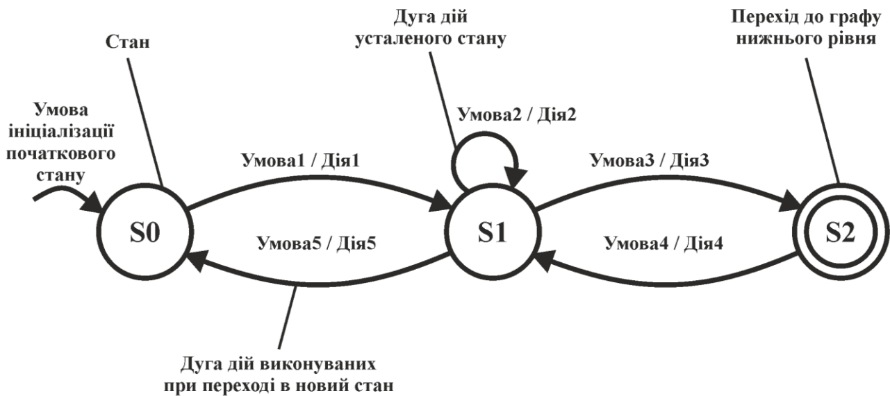
Рис. 1. Приклад графа станів
