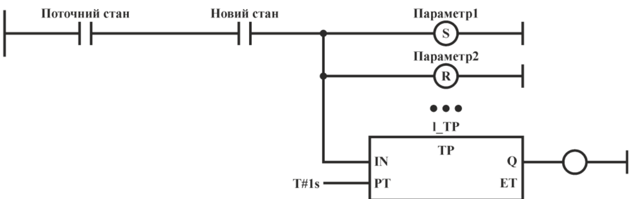
Рис. 3. Ланцюг дій
