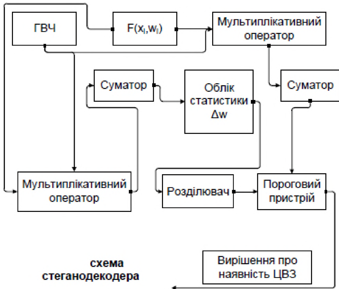
Рисунок 1.8 – Схеми стеганокодера і стеганодекодера згідно відомого підходу-прототипу [2, 32, 33]
