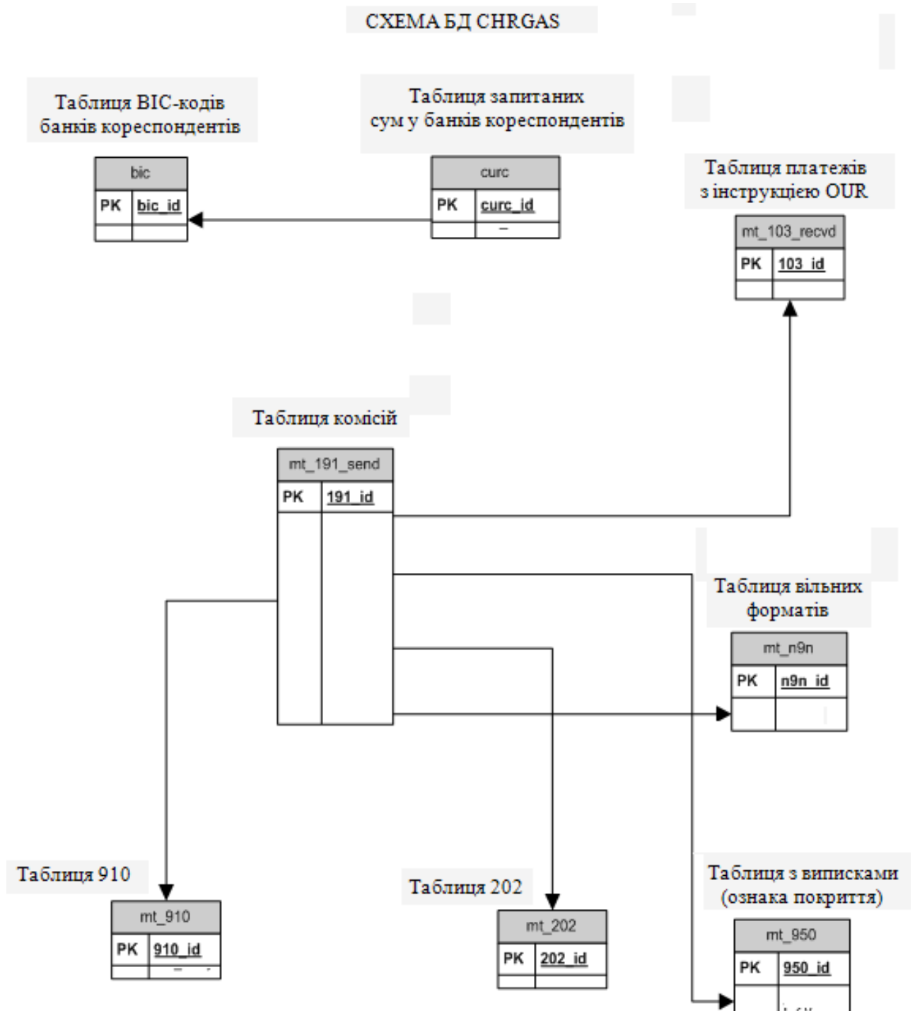
Рис. 2.1. Логічна структура бази даних
