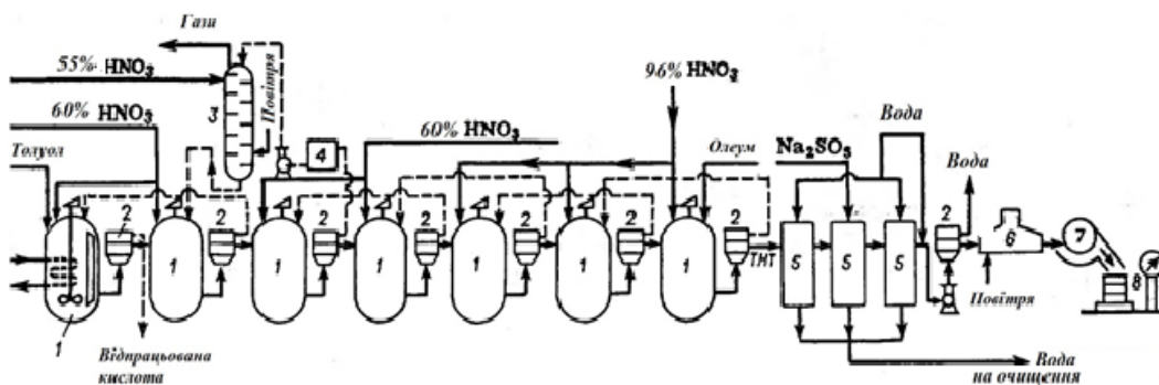
Рис. 1. Технологічна схема виробництва енергонасиченої речовини (тротилу):
