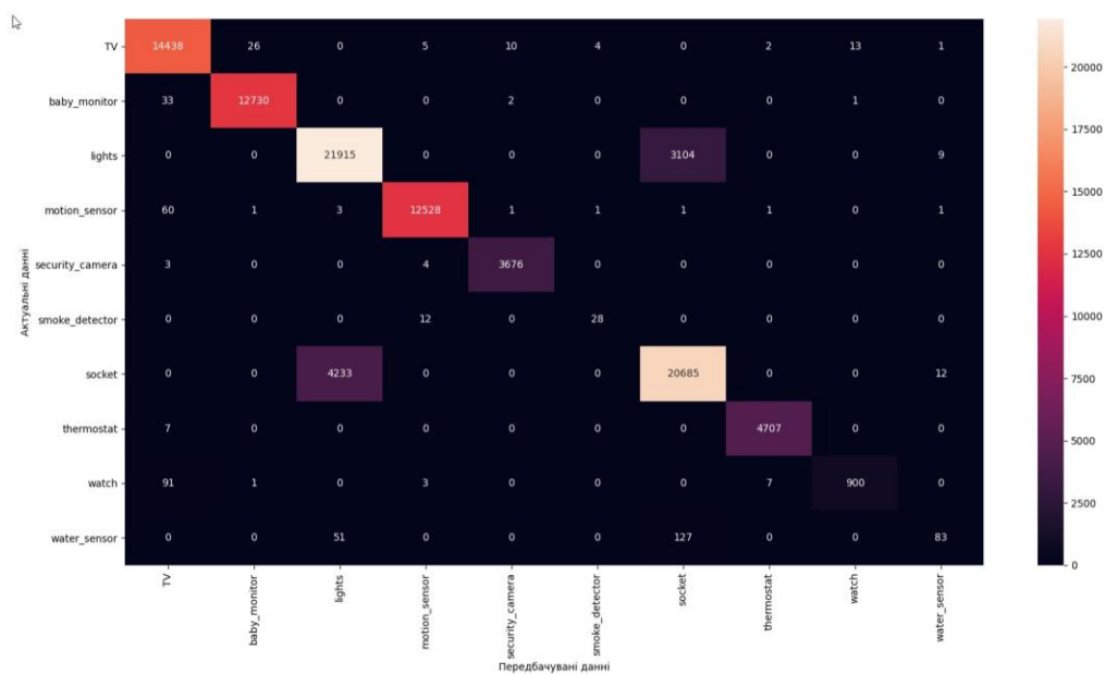
Рис. 3.3. Confusion Matrix для GradientBoosting
