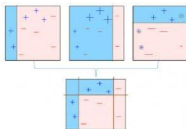
Рис. 2.4. Принцип роботи техніки Boosting (ч.2)
