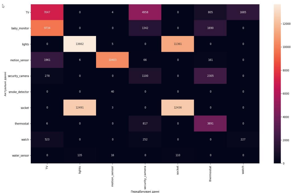
Рис. 3.4. Confusion Matrix для Ada Boosting
