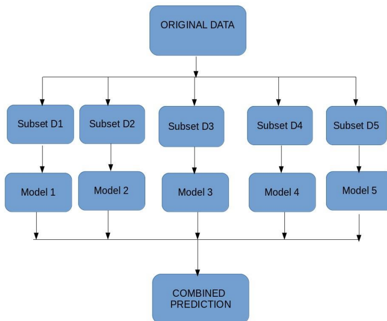
Рис. 2.2. Принцип роботи техніки Bagging(ч.2)
