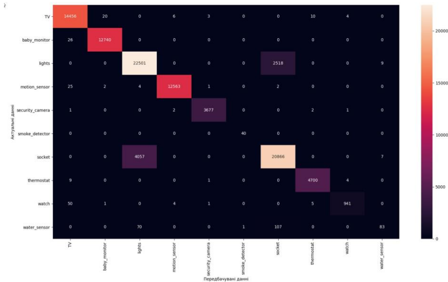
Рис. 3.2. Confusion Matrix для Bagging meta-estimator
