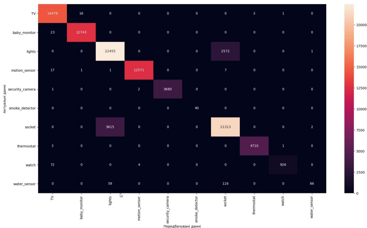
Рис. 3.1. Confusion Matrix для Random Forest
