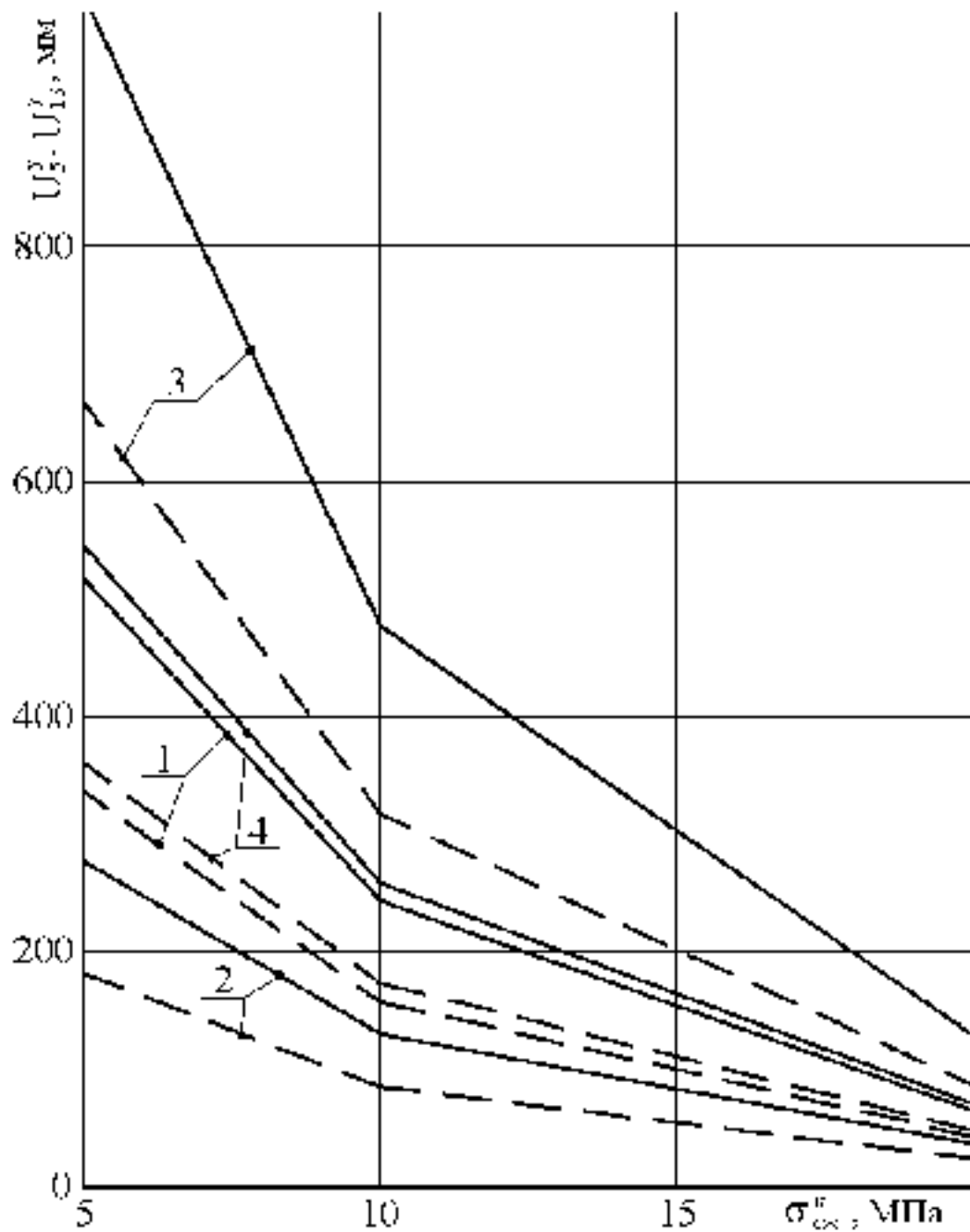
Рис. 3.11. Вертикальні переміщення U_5^y U_{13}^y зведення виробки в зоні проходу людей залежно від опору стискуванню \sigma_{csw}^k першого породного шару покрівлі :
