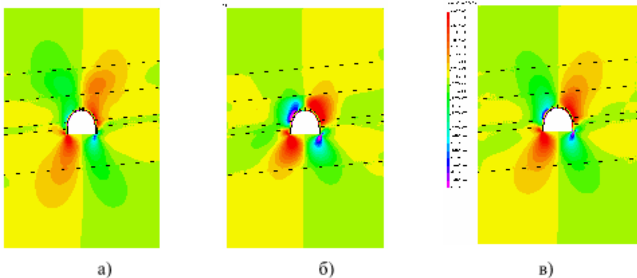
Рис. 3.6. Дотична напруга в моделі III при прослизанні породних шарів на глибині H = 200\text{м} : а - варіант А; б - варіант Б; в - варіант В
