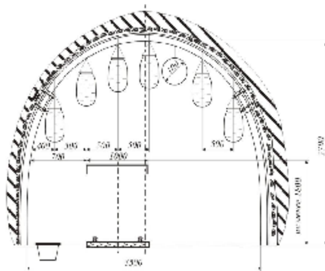
Рис. 3.13 — Схема установки водяного заслону з посудин ПБС-1
