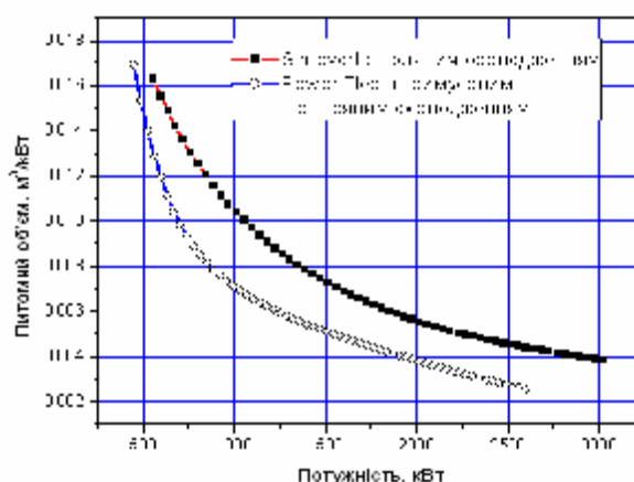
Рис. 5. Порівняння залежностей питомого об'єму високовольтних перетворювачів серії PowerFlex фірми Rockwell Automation з примусовим повітряним охолодженням (елементна база – SGCT) та серії Simovert фірми Siemens з водяним охолодженням (елементна база – IGBT)
