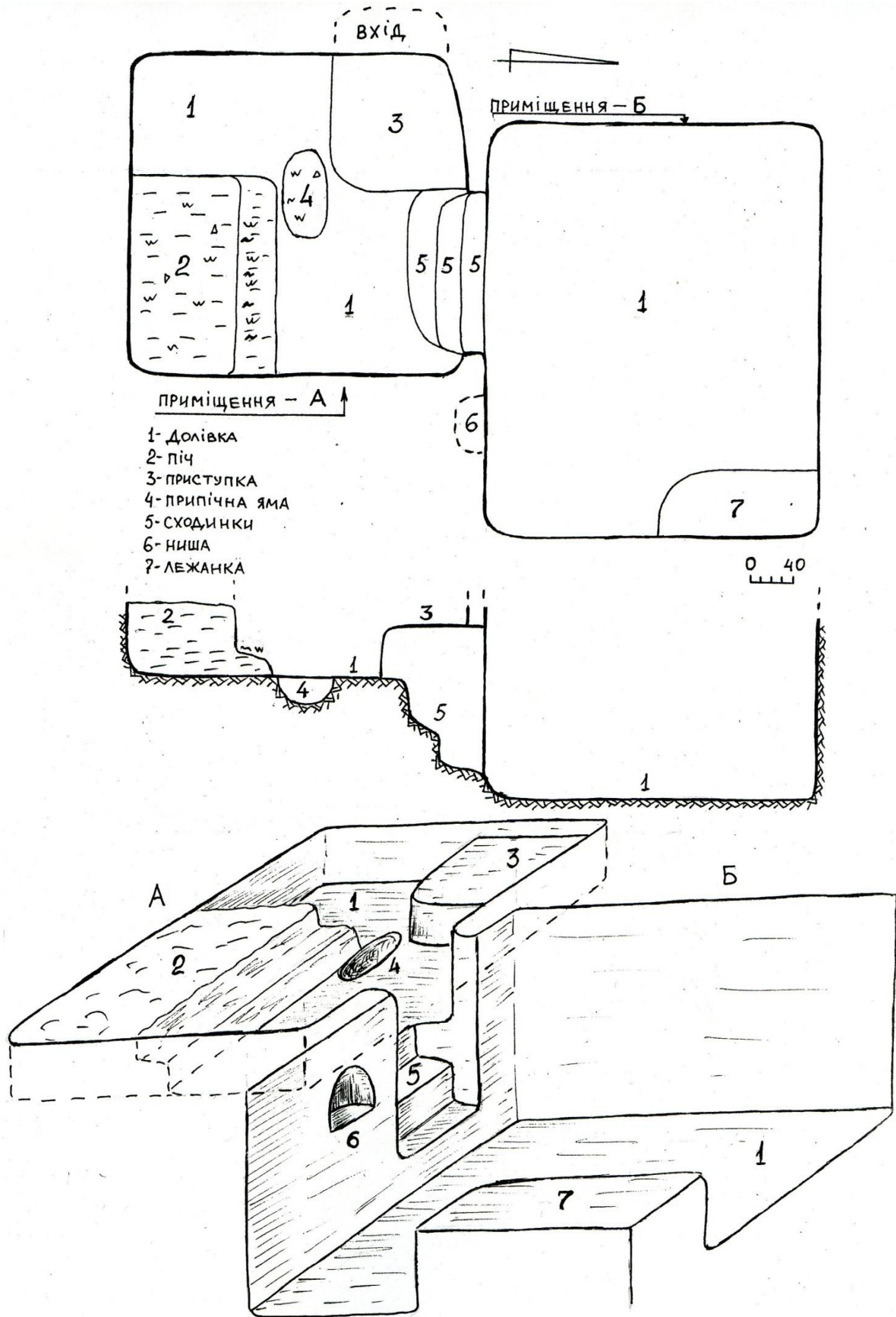
Рис. 1. Розкоп VIII. План та розріз землянки № 3 з козацької Самарі.
