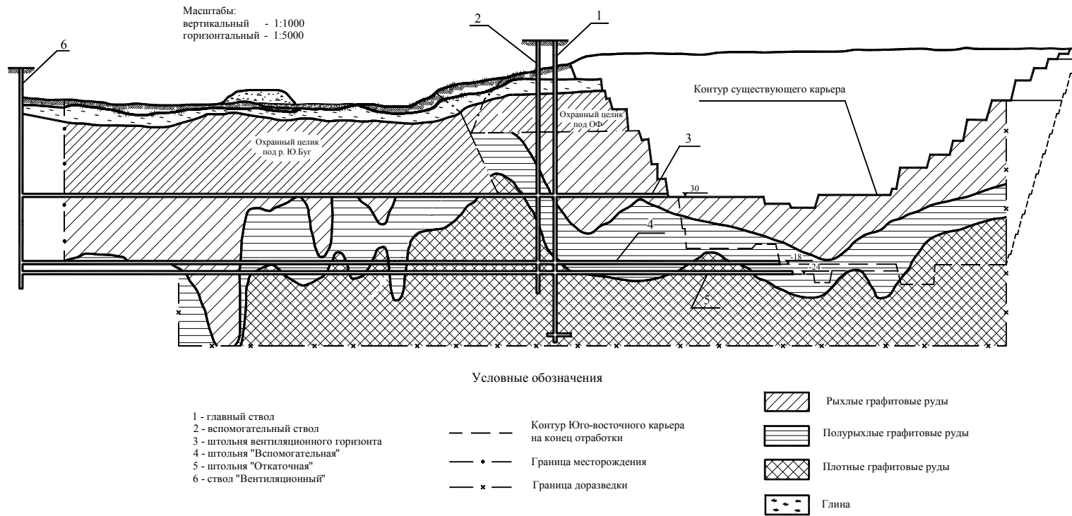
Рис. 2 .Схема вскрытия шахтного поля вертикальными стволами и штольнями
