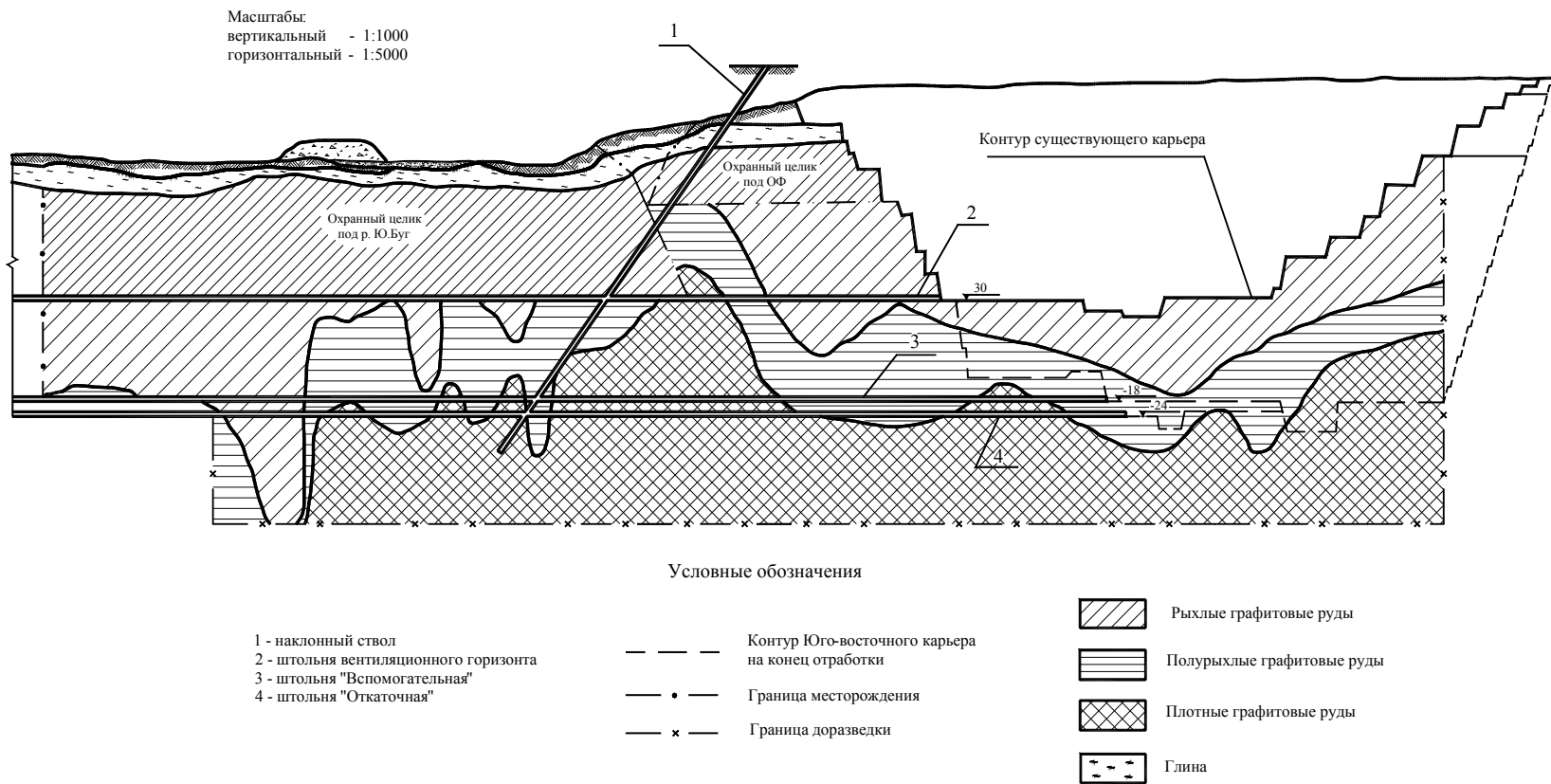
Рис. 1. Схема вскрытия шахтного поля наклонным стволом и штюлями
