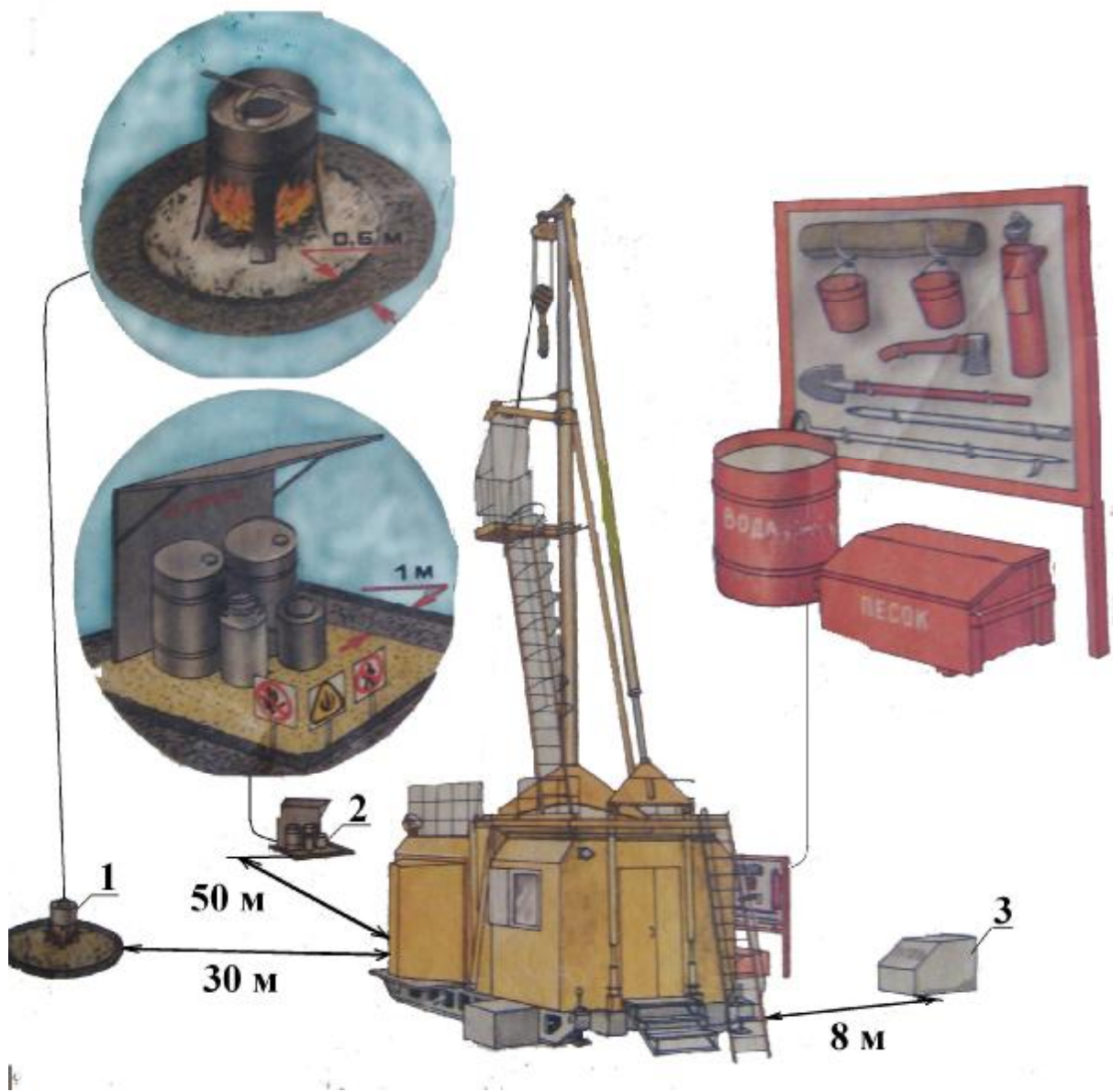
Рис. 5.7. Розміщення обладнання на буровій установці: 1 – місце для розігріву антивібраційного мастила, 2 – площадка для зберігання горюче-мастильних матеріалів, 3 – ящик для вугілля
