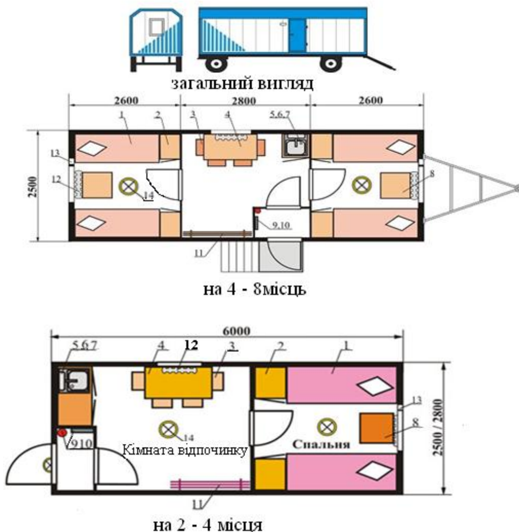
Рис. 2.3. Схеми вагон-будинків: 1 – спальні місця (полка верхня відкидна, полка нижня); 2 – шафа для одягу; 3 – табурет (4 шт.); 4 – стіл обідній; 5 – тумба з вбудованою мийкою; 6 – умивальник із підігрівом води; 7 – ємкість з пластика для води на 35 л; 8 – стіл-тумба; 9 – вогнегасник; 10 – електричний щиток; 11 – вішалка для верхнього одягу; 12 - вентилятор каналний; 14 - світильник
