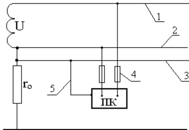
Рис. 4.6. Схема занулення ПК: 1 – фазний дріт; 2 – нульовий робочий дріт; 3 – нульовий захисний дріт; 4 – прилад струмового захисту; 5 – занулення.
