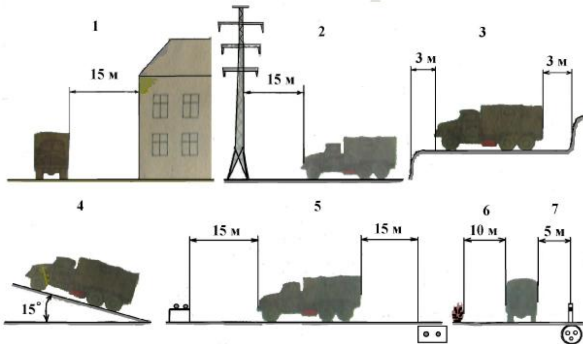
Рис. 3.19. Мінімальна відстань від джерела невибухового збудження до будівель (1), ліній електроживлення(2), обривів і крутих схилів (3), підземних і наземних трубопроводів (5), вогнищ (6), підземних кабельних ліній (7) і максимальних схилах (4)
