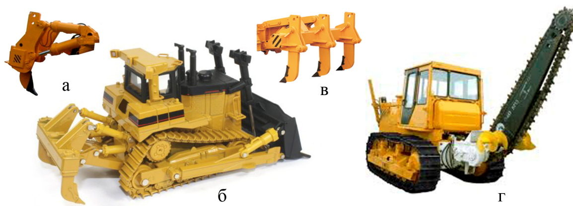
Рисунок 1 – Бульдозерно-розпушувальний агрегат з одно- (а), дво- (б) та багатозубим (в) розпушником; барова щілинонарізна машина (г)
