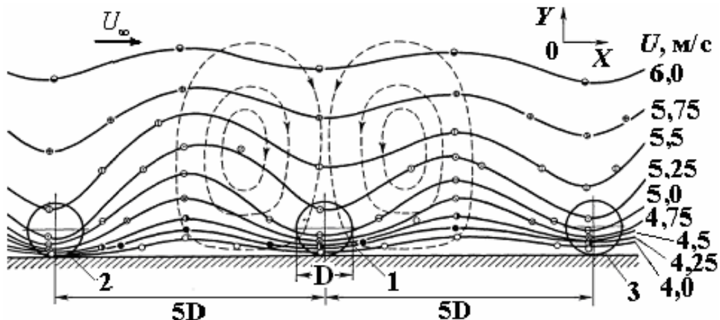
Рис. 1. Распределение результирующей скорости вязкой жидкости при обтекании шаров на плоской стенке (сплошная кривая) и вторичные течения в пограничном слое (штриховая линия): 1, 2, 3 – шары; D – диаметр шара, м; U – результирующая скорость вязкой жидкости, м/с; U_\infty – скорость набегающего потока, м/с [2, 3]
