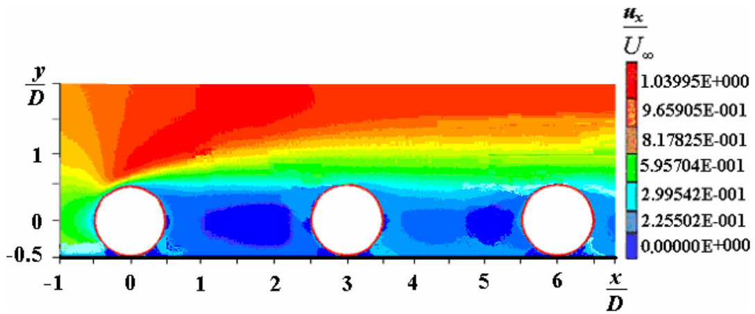
Рис. 5. Распределение продольной составляющей скорости вязкой жидкости, отнесенной к средней скорости набегающего потока
