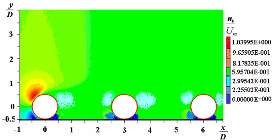
Рис. 6. Распределение поперечной составляющей скорости вязкой жидкости, отнесенной к средней скорости набегающего потока
