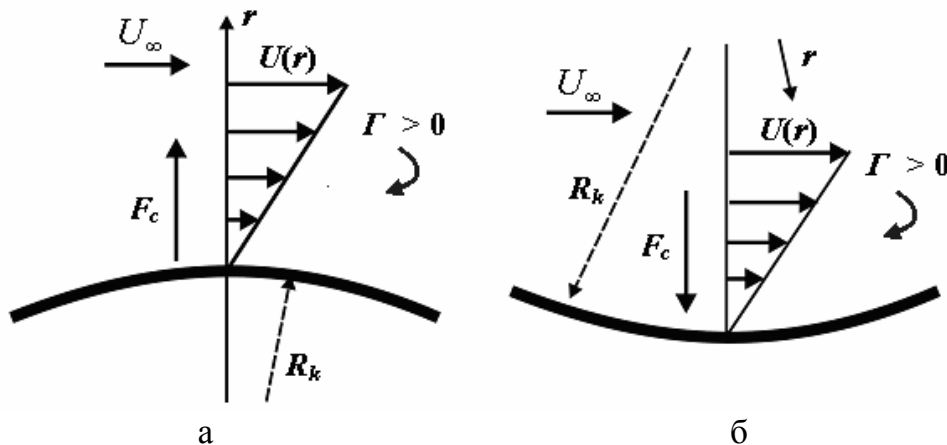
Рис. 2. Схемы течения вязкой жидкости в ламинарном пограничном слое на выпуклой (а) и вогнутой (б) поверхности: \Gamma = rU(r) – циркуляция скорости в вихре, \text{м}^2/\text{с} ; r – расстояние между центром кривизны поверхности и произвольной точкой потока, м; U(r) – распределение скорости вязкой жидкости в ламинарном пограничном слое, м/с; R_k – радиус кривизны поверхности, м; U_\infty – скорость набегающего потока, м/с; F_c – центробежная сила, Н
