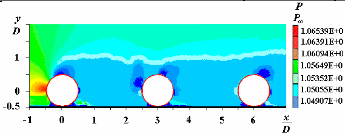
Рис. 4. Распределение давления вязкой жидкости, отнесенного к среднему давлению набегающего потока
