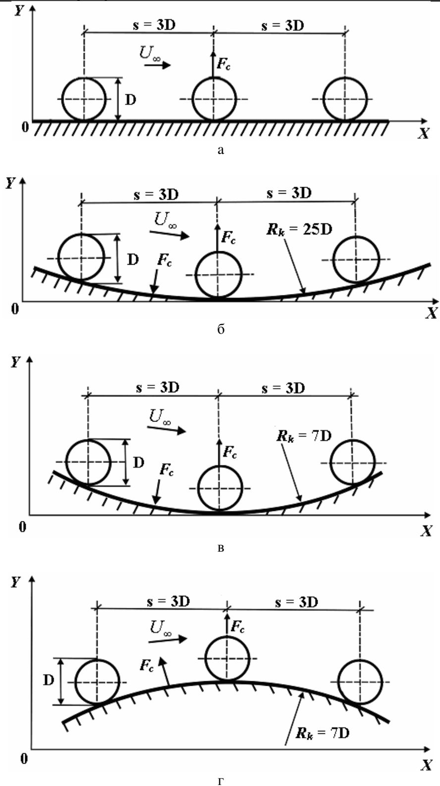
Рис. 3. Схеми обтекания потоком вязкой жидкости трех тандемных цилиндров, расположенных на горизонтальной (а), вогнутой (б, в) и выпуклой (г) стенках: R_k – радиус кривизны поверхности, м; U_\infty – скорость набегающего потока, м/с; F_c – центробежная сила, Н; D – диаметр цилиндра, м
