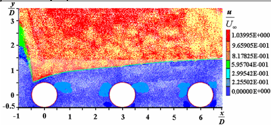
Рис. 7. Распределение результирующей скорости вязкой жидкости, отнесенной к средней скорости набегающего потока
