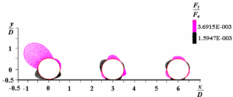
Рис. 11. Общий вид эпюры силы трения вязкой жидкости на поверхности цилиндров, отнесенной к средней величине силы трения на цилиндрической поверхности с единичной площадью ( F_s = \tau_0 S_0 \cos\theta , где \tau_0 – касательное напряжение на поверхности цилиндра [2], Па; S_0 = 1 – единичная площадь; \theta – угол между касательной к поверхности цилиндра и направлением средней скорости набегающего потока, град)
