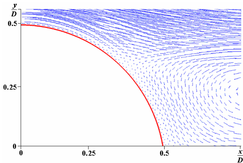
Рис. 8. Поле вектора результирующей скорости вязкой жидкости вблизи точки отрыва на цилиндре 1
