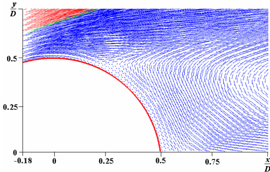
Рис. 10. Поле вектора результирующей скорости вязкой жидкости вблизи точки отрыва на цилиндре 3
