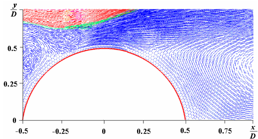
Рис. 9. Поле вектора результирующей скорости вязкой жидкости вблизи точки отрыва и присоединения на цилиндре 2
