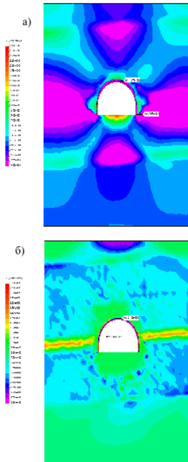
Рис. 3.15. Епюри розподілу горизонтальних напружень \sigma_x при знижених характеристиках міцності і підвищених деформаційних характеристиках всіх прилеглих породних шарів: а – H = 200\text{м} ; б – H = 600\text{м}
