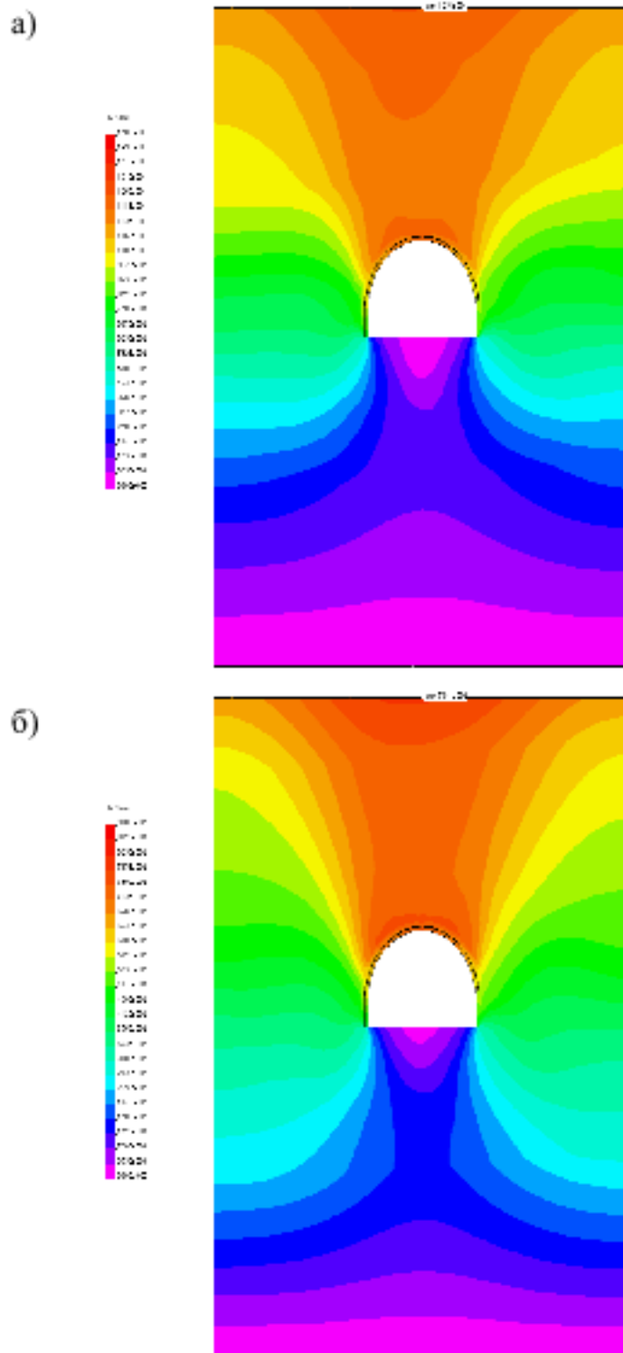
Рис. 3.10. Епюри повних переміщень при знижених характеристиках міцності всіх прилеглих породних шарів (див. Табл. 3.1) за варіантами їх деформаційних властивостей : а – №10; б – №18
