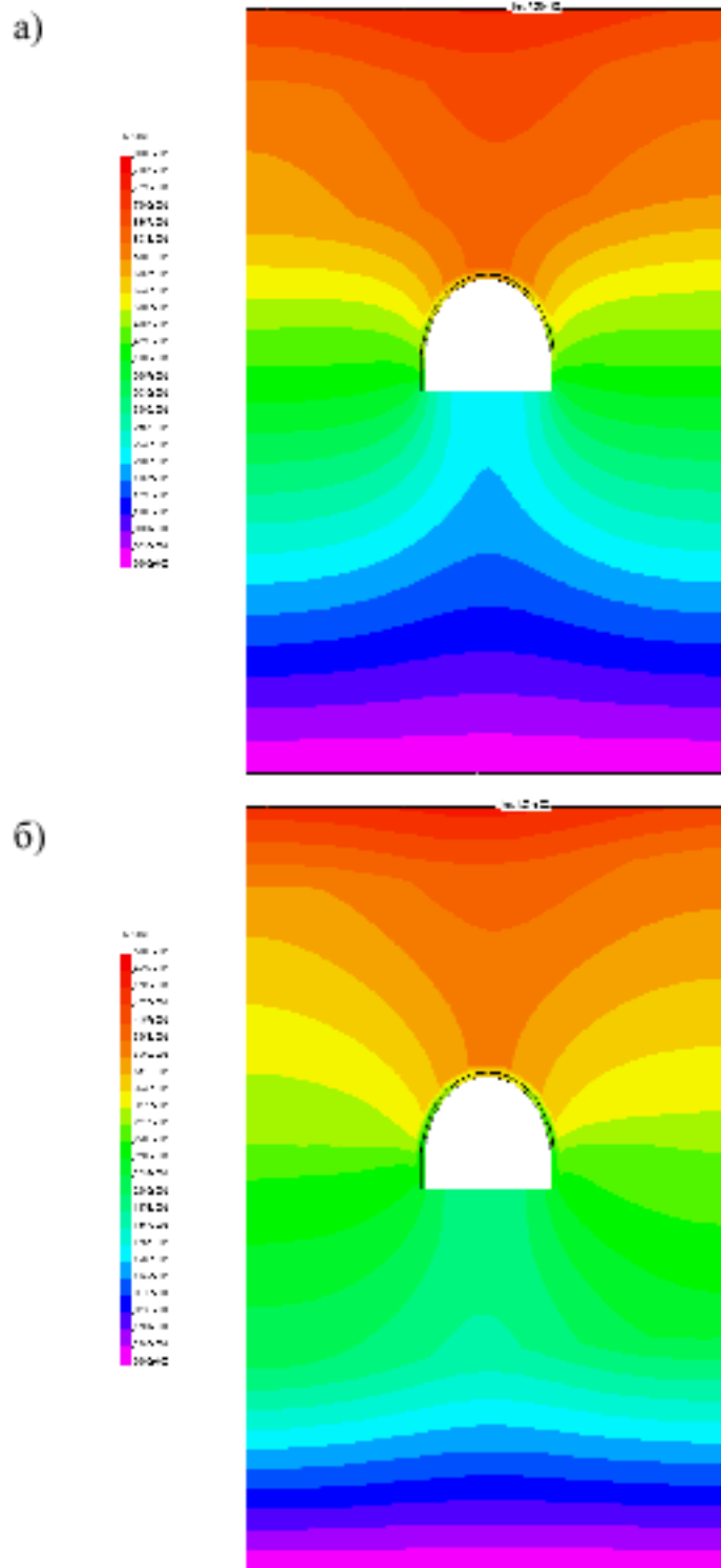
Рис. 3.11. Епюри повних переміщень при підвищених характеристиках міцності всіх прилеглих породних шарів (див. табл. 3.1) за варіантами їх деформаційних властивостей: а – №10; б – №18
