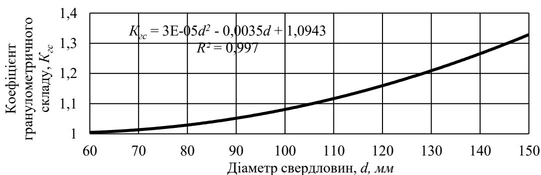
Рис. 5. Залежність величини коефіцієнта гранулометричного складу подрібненої руди захисного екрана K_{zc} від діаметра d глибоких свердловин, якими формується захисний екран: R^2 – достовірність апроксимації.
