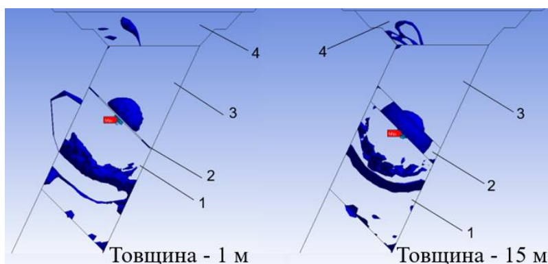
Рис. 2. Розповсюдження напружень вибухових хвиль у рудному масиві у вигляді ізоповерхні відповідно при товщині 1 м та 15 м захисного екрана: 1 – тіло магнетитового кварциту; 2 – захисний екран з відбитої розпушеної руди; 3 – бар'єрний цілик; 4 – кар'єр.
