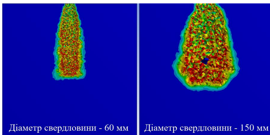
Рис. 4. Епюри подрібнення магнетитового кварциту у вигляді градієнтної кольорової діаграми на розрізі моделі по центру свердловини відповідно діаметром 60 мм та 150 мм і завдовжки 5 м після вибуху
