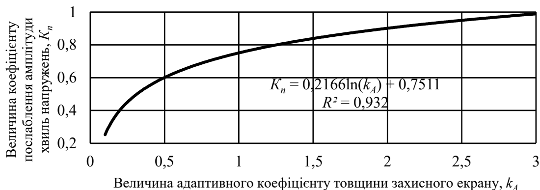
Рис. 3. Залежність величини коефіцієнту послаблення K_n амплітуди хвиль напружень під час їхнього поширення в екранувальному шарі захисного екрана з подрібненої руди від адаптивного коефіцієнту k_A товщини захисного екрана: R^2 – достовірність апроксимації
