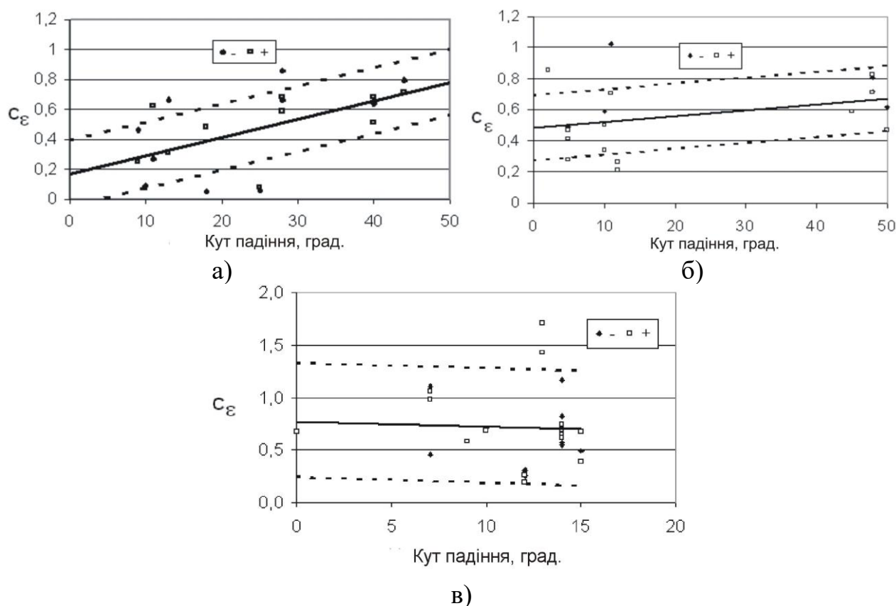
Рис. 3. Графіки коефіцієнтів максимальних горизонтальних деформацій: а – висока ступінь метаморфізму (марки вугілля Т, А); б – середня ступінь метаморфізму (марки вугілля Ж, К, ОС); в – низький ступінь метаморфізму (марки вугілля Д, Г)
