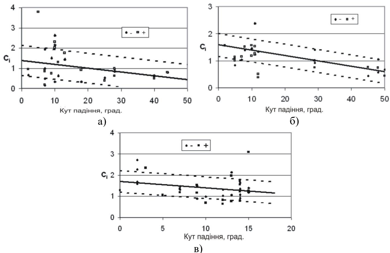
Рис. 1. Графіки коефіцієнтів максимальних нахилів: а – високий ступінь метаморфізму (марки вугілля Т, А); б – середній ступінь метаморфізму (марки вугілля Ж, К, ОС); в – низький ступінь метаморфізму (марки вугілля Д, Г).
