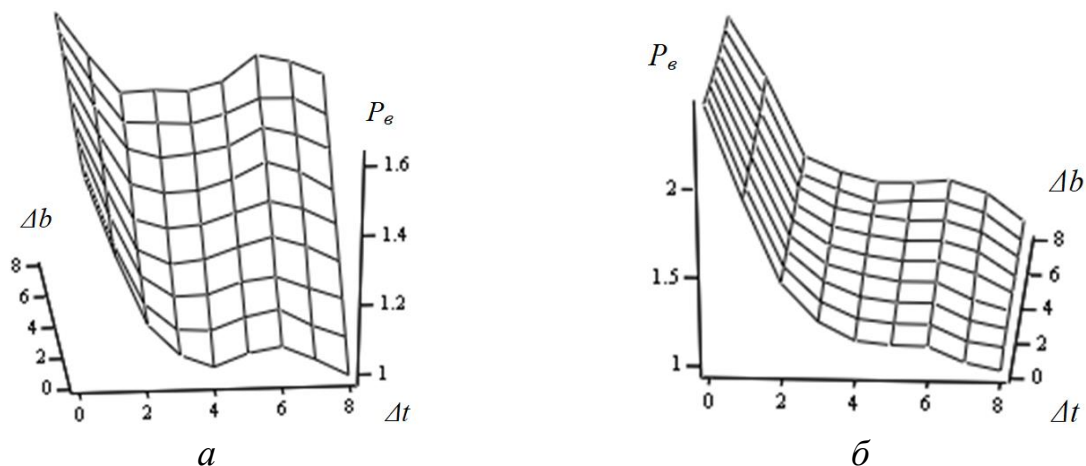
Рис. 8. Значення сил для каната з тросів умовно круглого перерізу, віднесених до сил стискання для каната з урахуванням його побудови з окремих стренг для різних значень параметрів \Delta t та \Delta b : a – відповідно до рисунку 1, a ; б – відповідно до рисунку 1, б
