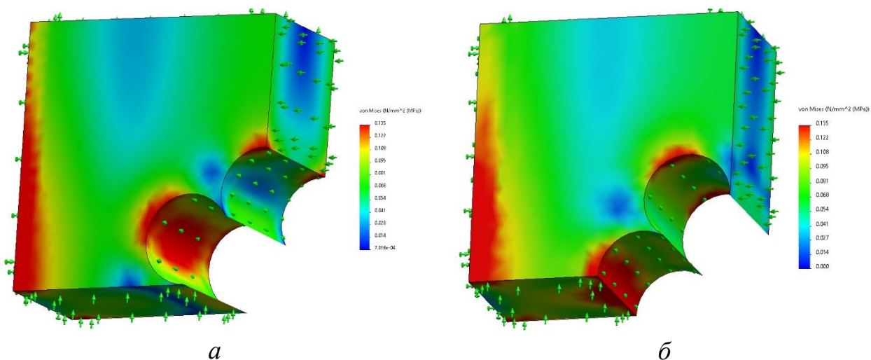
Рис. 13. Напруження у чверті гумового прошарку від зсуву за зближення тросів каната; a – відповідно до рисунку 1, a ; б – відповідно до рисунку 1, б
