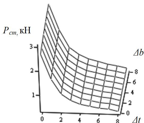
Рис. 6. Середні значення сил стискання P_{cm} для каната за різних значень параметрів \Delta t та \Delta b
