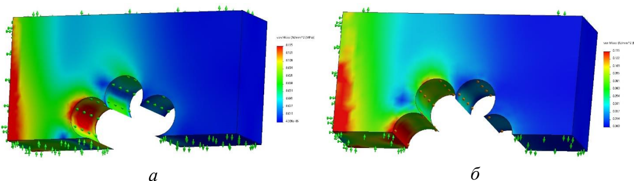
Рис. 14. Напруження у половині гумового прошарку від зсуву за зближення тросів каната; а – відповідно до рисунку 1, а ; б – відповідно до рисунку 1, б
