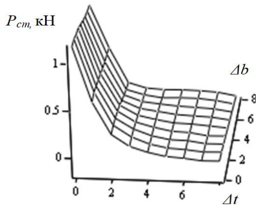
Рис. 5. Різниця сил стискання P_{cm} для каната за різних значень параметрів \Delta t та \Delta b за розташування стренг каната відповідно до рисунків 1, a – 1, б
