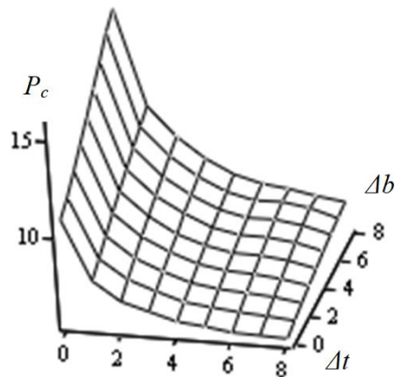
Рис. 21. Значення відносних сил зсуву P_c – відношення сил зсуву гумового прошарку прямокутного профілю до відповідних сил в прошарках для каната з реальною (некруглою) формою перерізів, зображеного на рисунку 1, а для різних значень параметрів \Delta t та \Delta b
