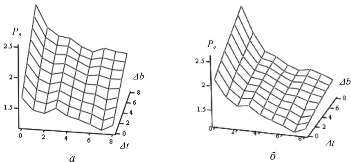
Рис. 11. Значення сил для каната з тросів умовного прямокутного перерізу, віднесених до сил стискання для каната з урахуванням його побудови з окремих стренг для різних значень параметрів \Delta t та \Delta b : a – відповідно до рисунку 1, а ; б – відповідно до рисунку 1, б
