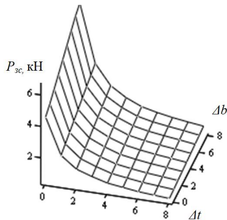
Рис. 20. Значення сил зсуву P_{zc} для каната з тросів умовного прямокутного перерізу для різних значень параметрів \Delta t та \Delta b
