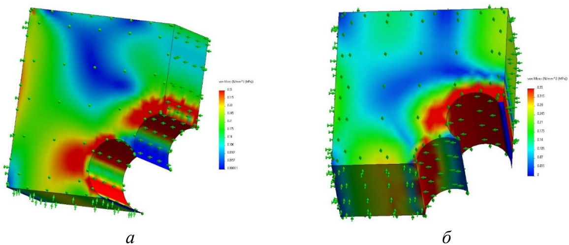
Рис. 2. Напруження у чверті гумового прошарку від стиску за зближення тросів каната; а – відповідно до рисунку 1, а ; б – відповідно до рисунку 1, б
