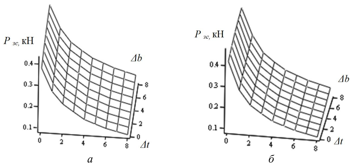
Рис. 15. Значення сил зсуву P_{zc} для канатів за різних значень параметрів \Delta t та \Delta b за розташування стренг каната: а – відповідно до рисунку 1, а ; б – відповідно до рисунку 1, б
