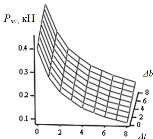
Рис. 17. Середнє значення сил зсуву P_{zc} для каната за різних значень параметрів \Delta t та \Delta b за розташування стренг каната відповідно до рисунків 1, а – 1, б
