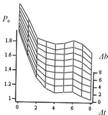
Рис. 9. Середні значення сил для каната з тросів умовно круглого перерізу, віднесених до сил стискання для каната з урахуванням його побудови з окремих стренг для різних значень параметрів \Delta t та \Delta b
