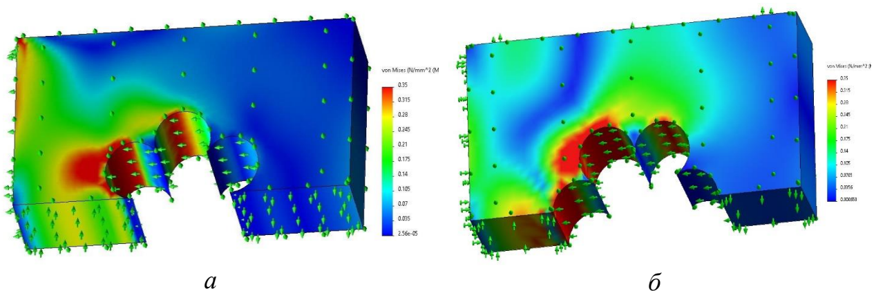
Рис. 3. Напруження у половині гумового прошарку від стиску за зближення тросів каната; а – відповідно до рисунку 1, а ; б – відповідно до рисунку 1, б
