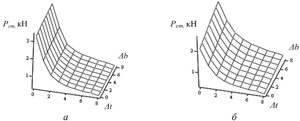
Рис. 4. Значення сили стискання P_{cm} для каната за різних значень параметрів \Delta t та \Delta b за розташування стренг каната: a – відповідно до рисунку 1, a ; б – відповідно до рисунку 1, б
