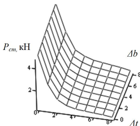
Рис. 7. Значення сил стискання P_{cm} для каната з тросами умовно круглого перерізу за різних значень параметрів \Delta t та \Delta b
