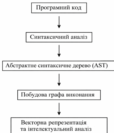
Рисунок 1 – Схема методу інтелектуального аналізу програмного коду
