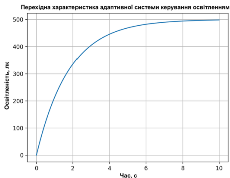
Рисунок 1 – Перехідний процес стабілізації освітленості
