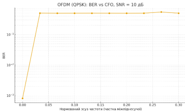
Рисунок 1 – Вплив нормованого частотного зсуву (CFO) на BER у системі OFDM.
