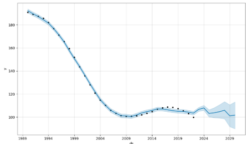
Рисунок 2 – Прогноз динаміки показника children за моделлю Prophet
