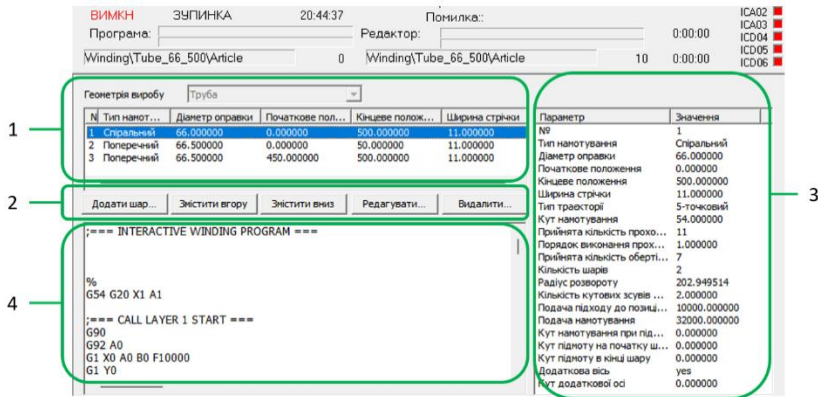
Рисунок 1 – Вікно для проектування структури шарів труби
