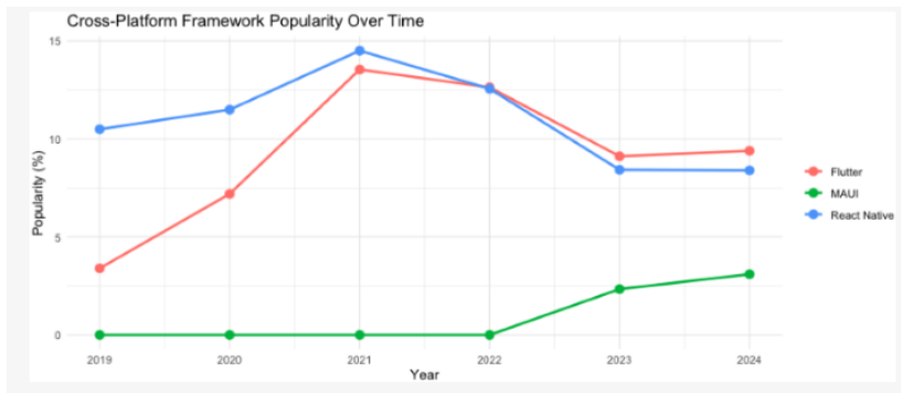
Рис 1 - Популярність кросплатформних фреймворків серед розробників
