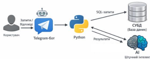
Рисунок 1. Інтеграція Telegram-бота, Python, бази даних і AI для автоматизованих систем
