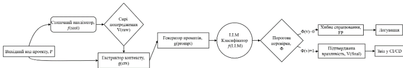
Рисунок 1 –Модель процесу валідації результатів статичного аналізу за допомогою LLM
