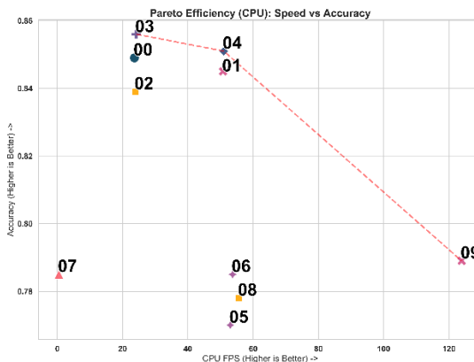
Рис. 1. Парето-фронт ефективності методів компресії для ResNet на системі з обмеженим енергоспоживанням (CPU).
