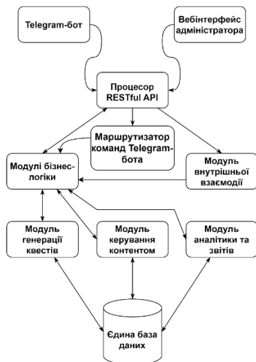
Рисунок 1 – Архітектура системи генерації персоналізованих квестів
