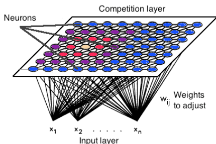
Рисунок 1 – структурна схема самоорганізовуваної карти Кохонена[4]
