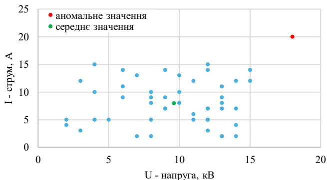
Рисунок 1 – Визначення аномального режиму за інтегральним показником відхилення D_M(\tau)
