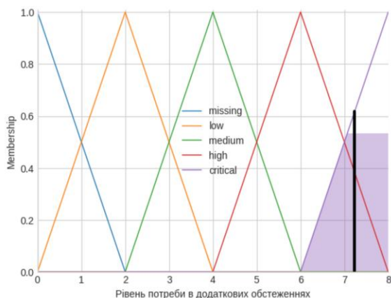
Рисунок 3 – Результат роботи програми на графіку
