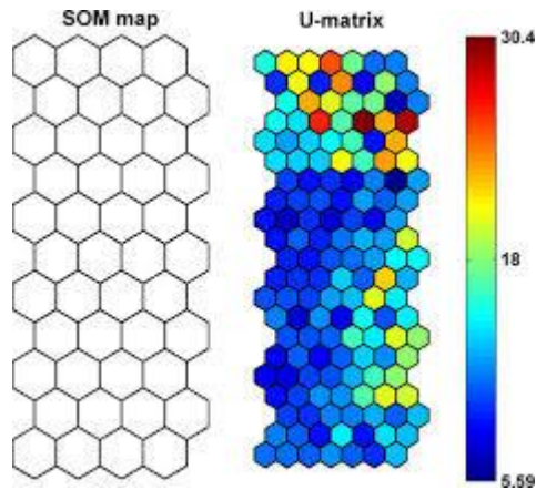
Рисунок 2 – вигляд самоорганізовуваної карти Кохонена та модель U-matrix[5]
