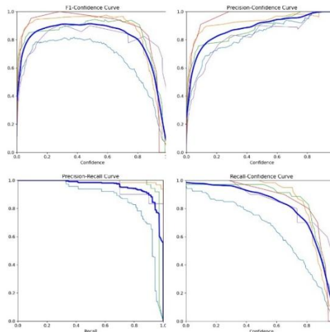
Рисунок 1 – Криві залежності точності, повноти та F1-міри
