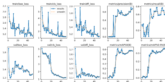
Рисунок 1 – Динаміка зміни функції втрат та основних метрик під час навчання моделі YOLOv8
