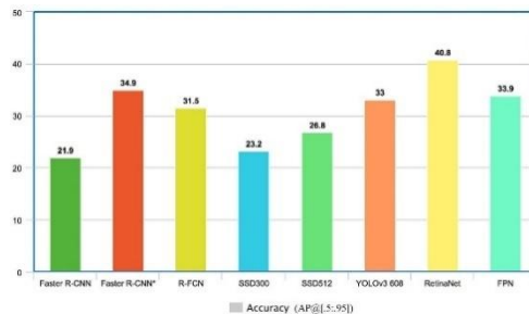
Рисунок 1 – Точність розпізнавання різних алгоритмів [1].
