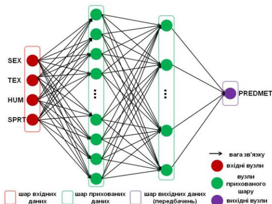
Рисунок 1 – Узагальнена архітектура інформаційної системи прогнозування освітнього вибору
