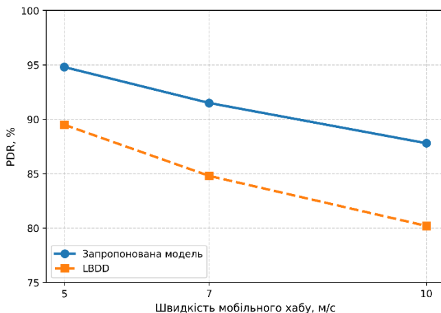
Рисунок 1 – Залежність PDR від швидкості руху хабу
