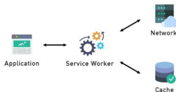
Рисунок 2 – Архітектурна модель роботи PWA
