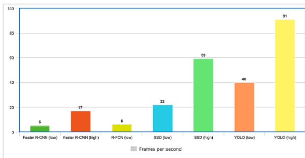
Рисунок 2 – Швидкість розпізнавання різних алгоритмів [1].
