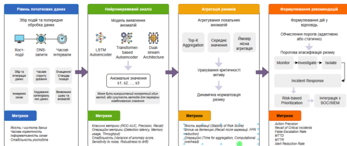
Рисунок 1—Архітектура гібридної системи підтримки прийняття рішень
