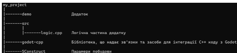
Рисунок 1 – Загальна структура додатку
