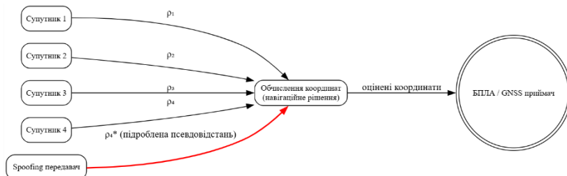
Рисунок 1 – Вплив spoofing-атаки на навігаційні вимірювання GNSS приймача
