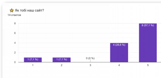
Рисунок 2 – Результати опитування
