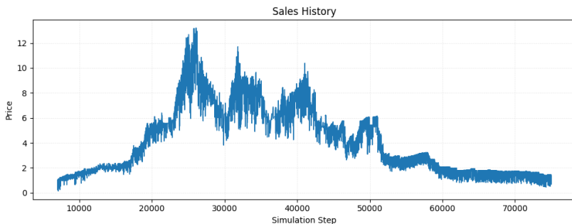
Рисунок 1 – Графік продажів для однієї з симуляцій
