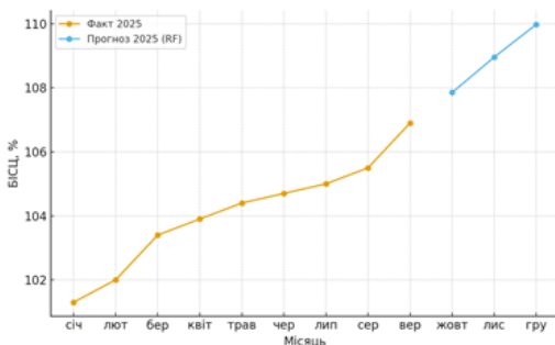
Рисунок 1 – Фактичні та прогнозні значення базового індексу споживчих цін України у 2025 році
