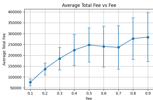
Рисунок 3 – Залежність суми заробітку з комісійних від ставки комісії, для одного з експериментів
