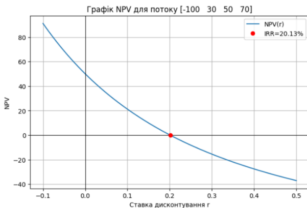
Рисунок 1 – Графічна залежність функції NPV від ставки дисконтування та визначення точки IRR
