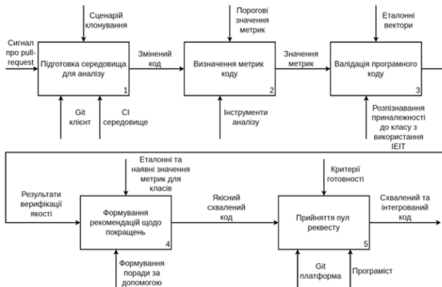
Рисунок Помилка! У документі відсутній текст указанного стилю.1– Функціональна схема СППР для верифікації якості ПЗ
