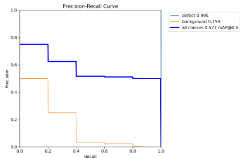
Рисунок 2 – Precision–Recall крива для моделі детекції сторонніх об’єктів
