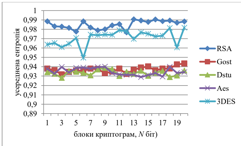
Рисунок 2. Результати досліджень усередненої ентропії блоків криптограм
