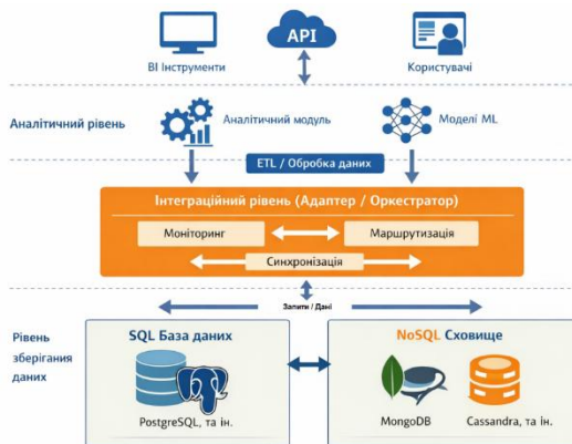
Рисунок 1 – Архітектура гібридної системи
