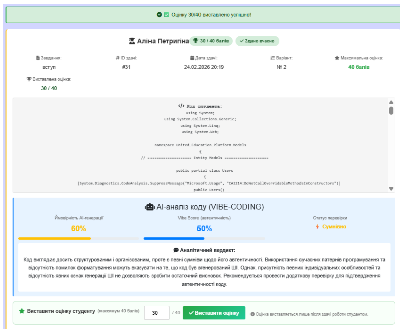
Рисунок 3 – Сторінка перевірки роботи студента та виставлення оцінки викладачем
