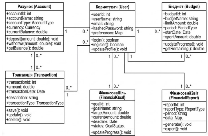
Рисунок 1 – Діаграма класів
