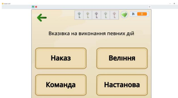
Рисунок 2 – Вікторина
