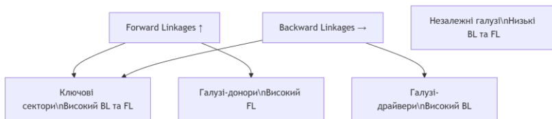
Рисунок 2 – Класифікація галузей за індексами міжгалузових зв'язків
