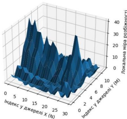
Рис. 1. Поверхня локальних розбіжностей між двома джерелами даних
