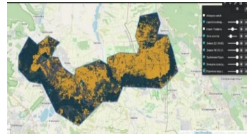
Рис. 2. - Втрати лісового покриву (207.10 км 2 ) у Серебрянському лісі.
