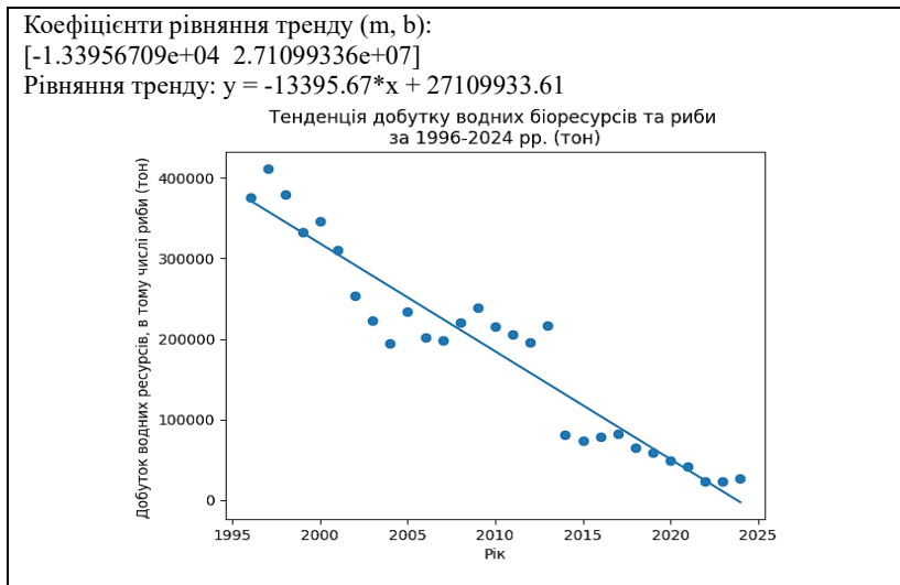
Рисунок 1. Результати реконструкції динаміки добутку водних біоресурсів та риби в Україні за 1996-2024 рр. (тон)
