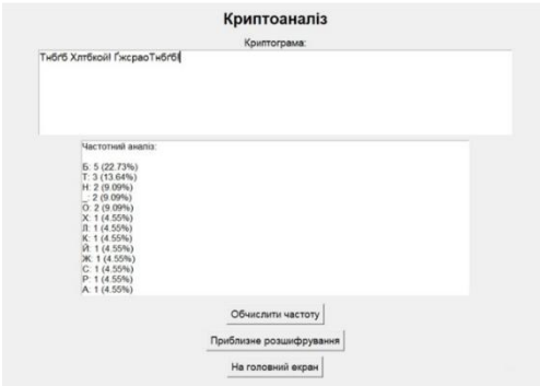
Рисунок 4 – Частотний аналіз
