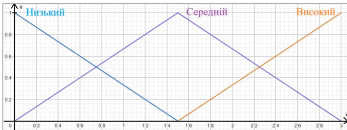
Рисунок 1 – Графік функції належності для термів лінгвістичної змінної "Рівень невизначеності діагнозу за оцінкою лікаря"
