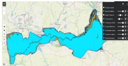
Рис. 3. - Втрата водної поверхні (1530.60 км 2 ) Каховського водосховища.
