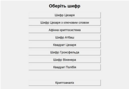
Рисунок 2 – Головний екран
