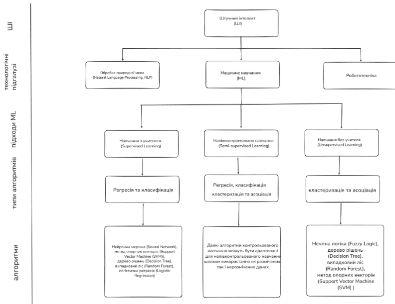
Рисунок 1 - Класифікація ШІ технологій
