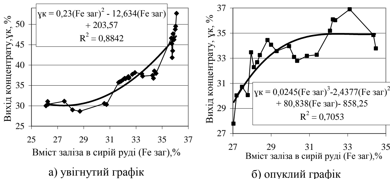
Рис. 2. Залежність виходу концентрату від вмісту заліза у сирій руді
