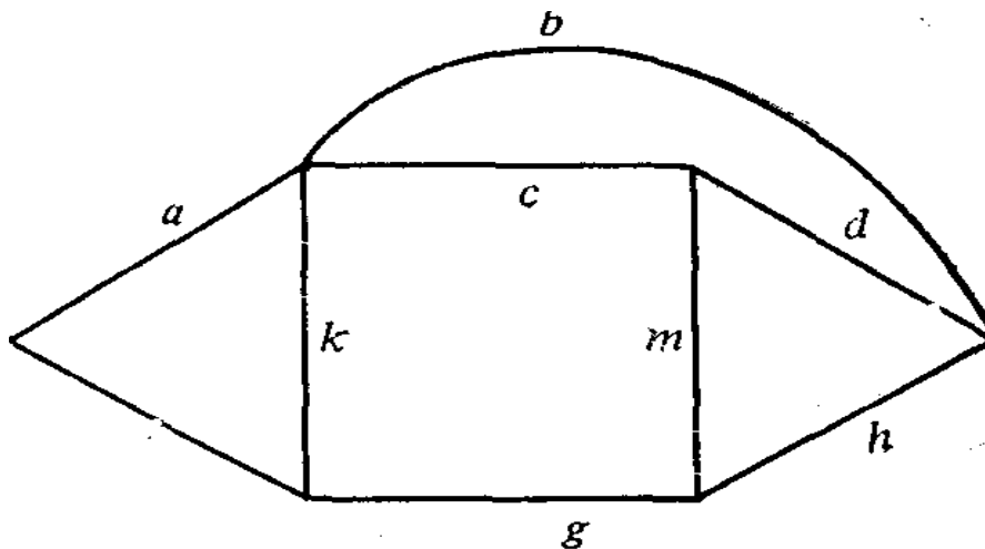
Рисунок 2.4 - Приклад мережі для розрахунку надійності по повній сукупності шляхів, де R_i=1-R_1 аналогічно (1.16).
